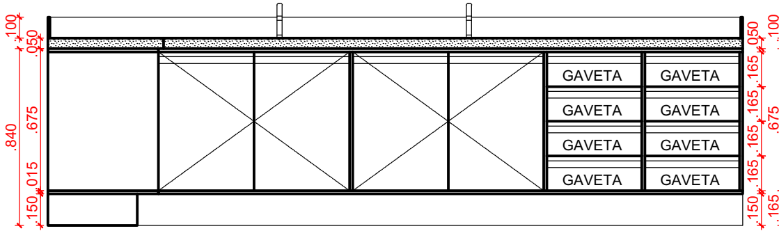
VISTA LATERAL
