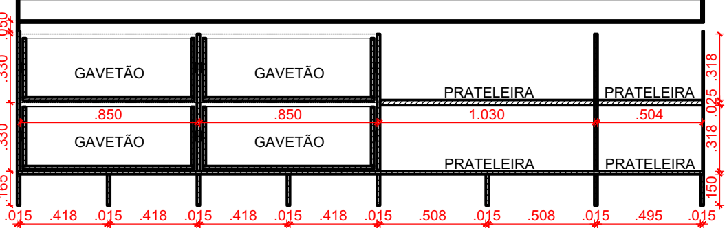
VISTA LATERAL
