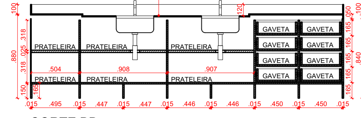
CORTE BB
