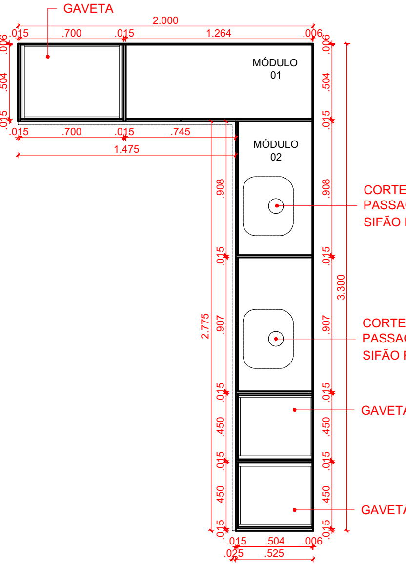
VISTA SUPERIOR - MÓVEL
