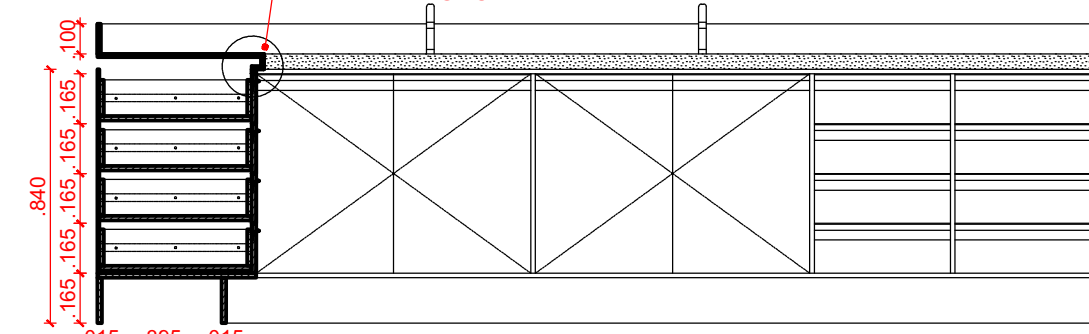
CORTE CC
