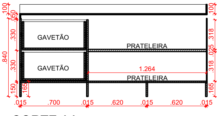
CORTE AA
