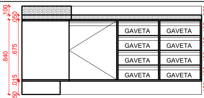
VISTA LATERAL
