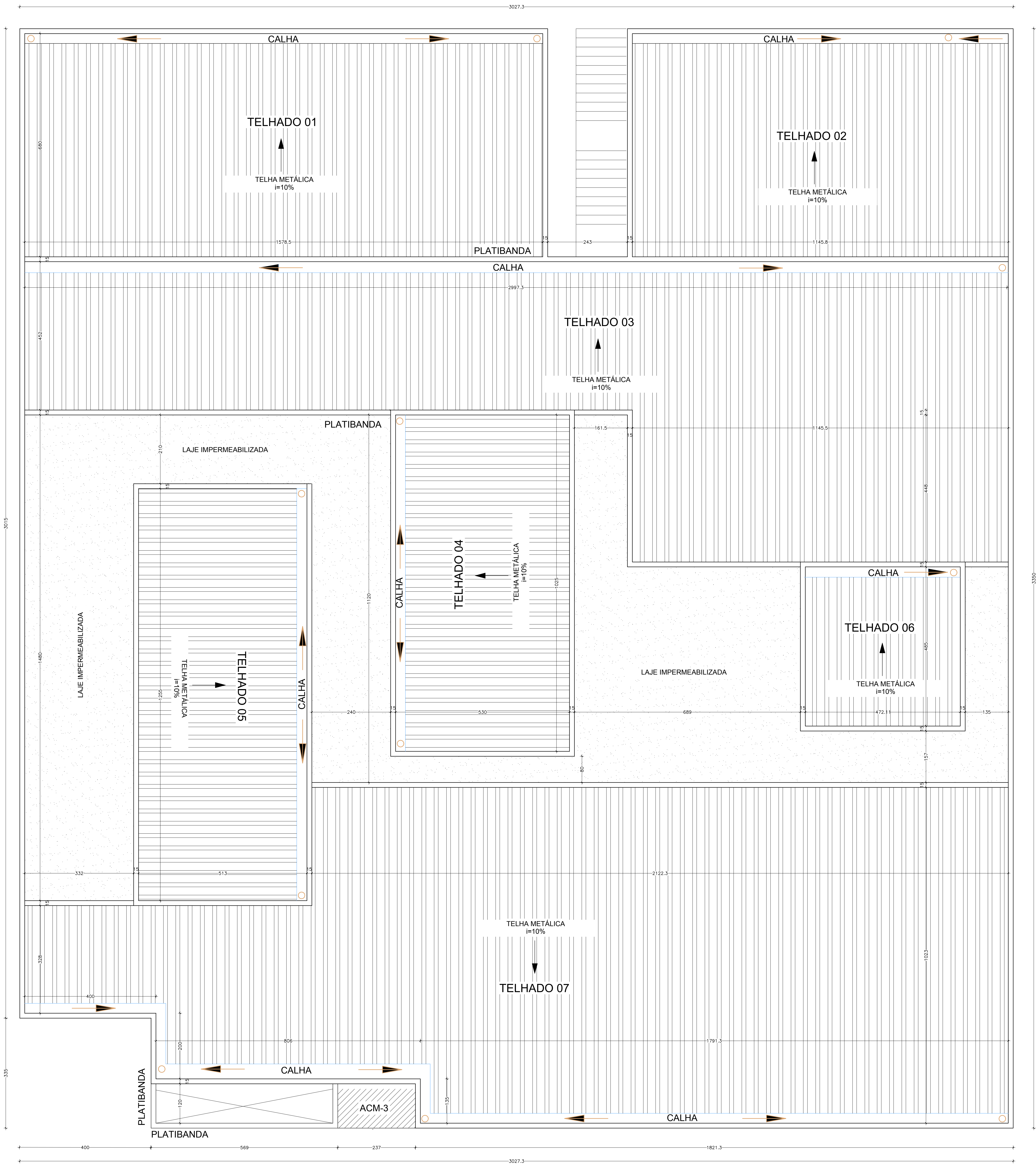
PLANTA GERAL DA COBERTURA ESCALA: 1:50
