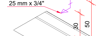
Detalhe HID-3 Escala 1:25
