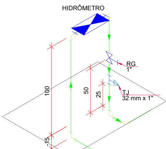
Detalhe HID-1 Escala 1:25
