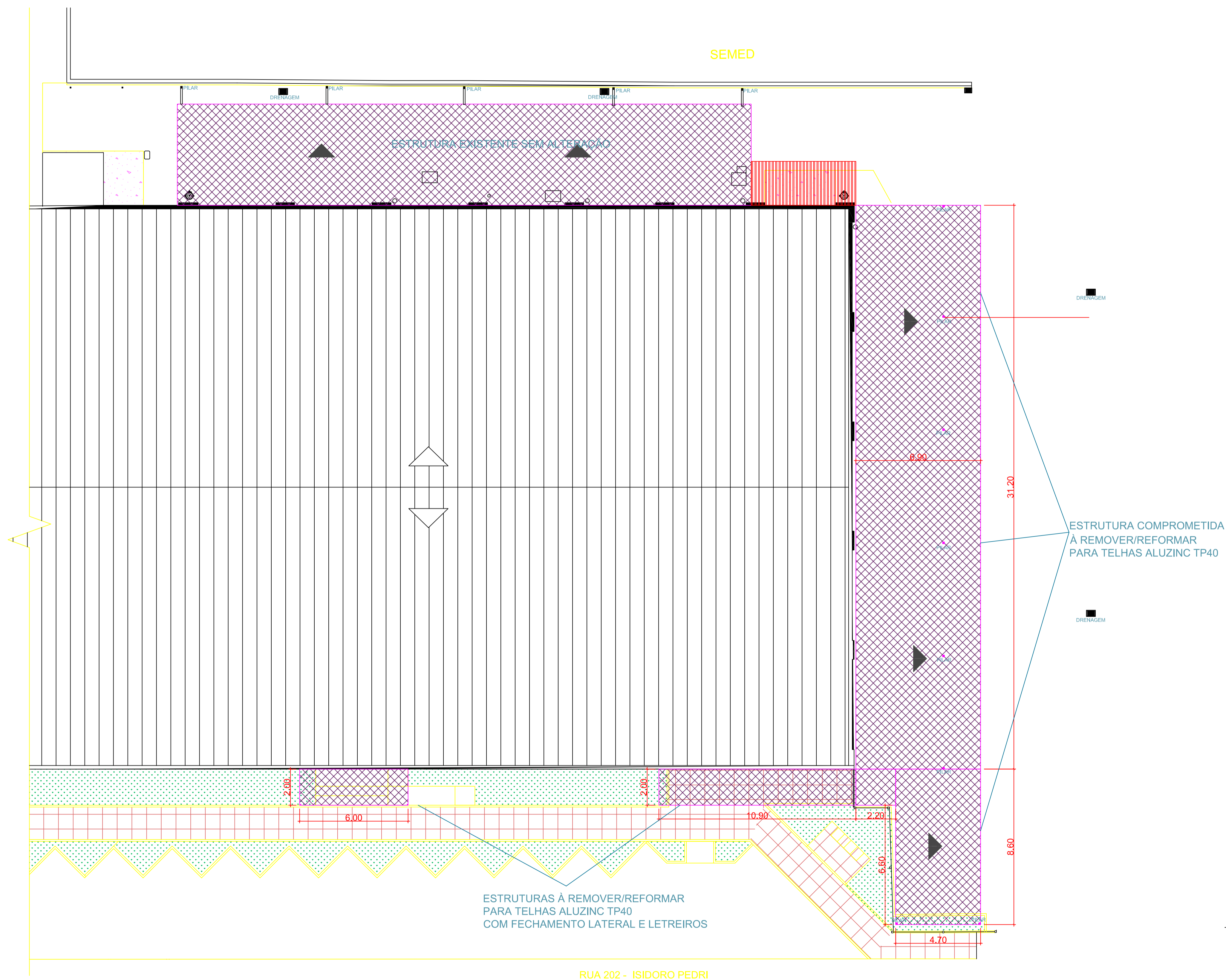
1 PLANTA BAIXA - Situação atual ESCALA 1:125
