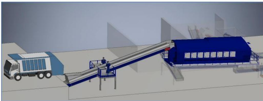
Figura 2: Alimentação, Triagem Manual e Peneira Giratória
