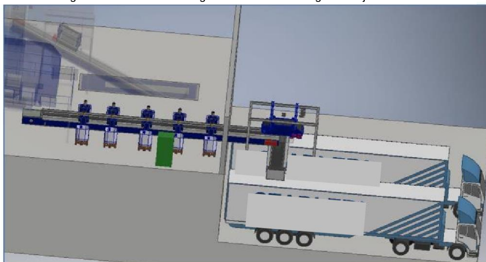
Figura 4: Processo de Triagem Manual e Descarga de Rejeitos
