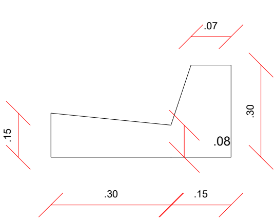
PLANTA DETALHE - MEIO-FIO E SARJETA
