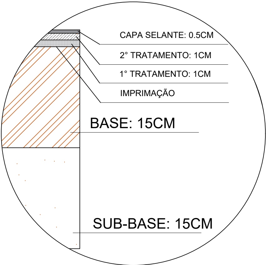
DETALHE TRANSVERSAL DO PAVIMENTO
