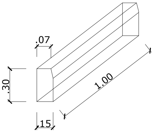
DETALHE MEIO FIO
