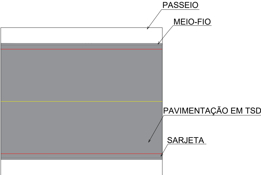
PLANTA DETALHE - PAVIMENTAÇÃO EM TRATAMENTO SUPERFICIAL DUPLO
