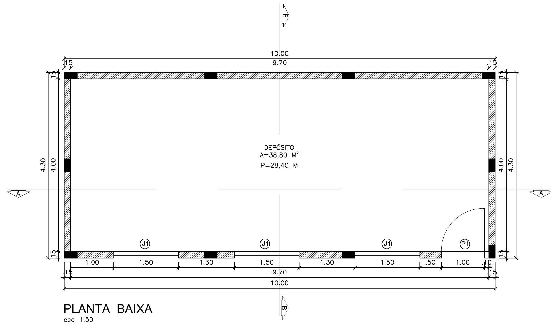
PLANTA BAIXA
