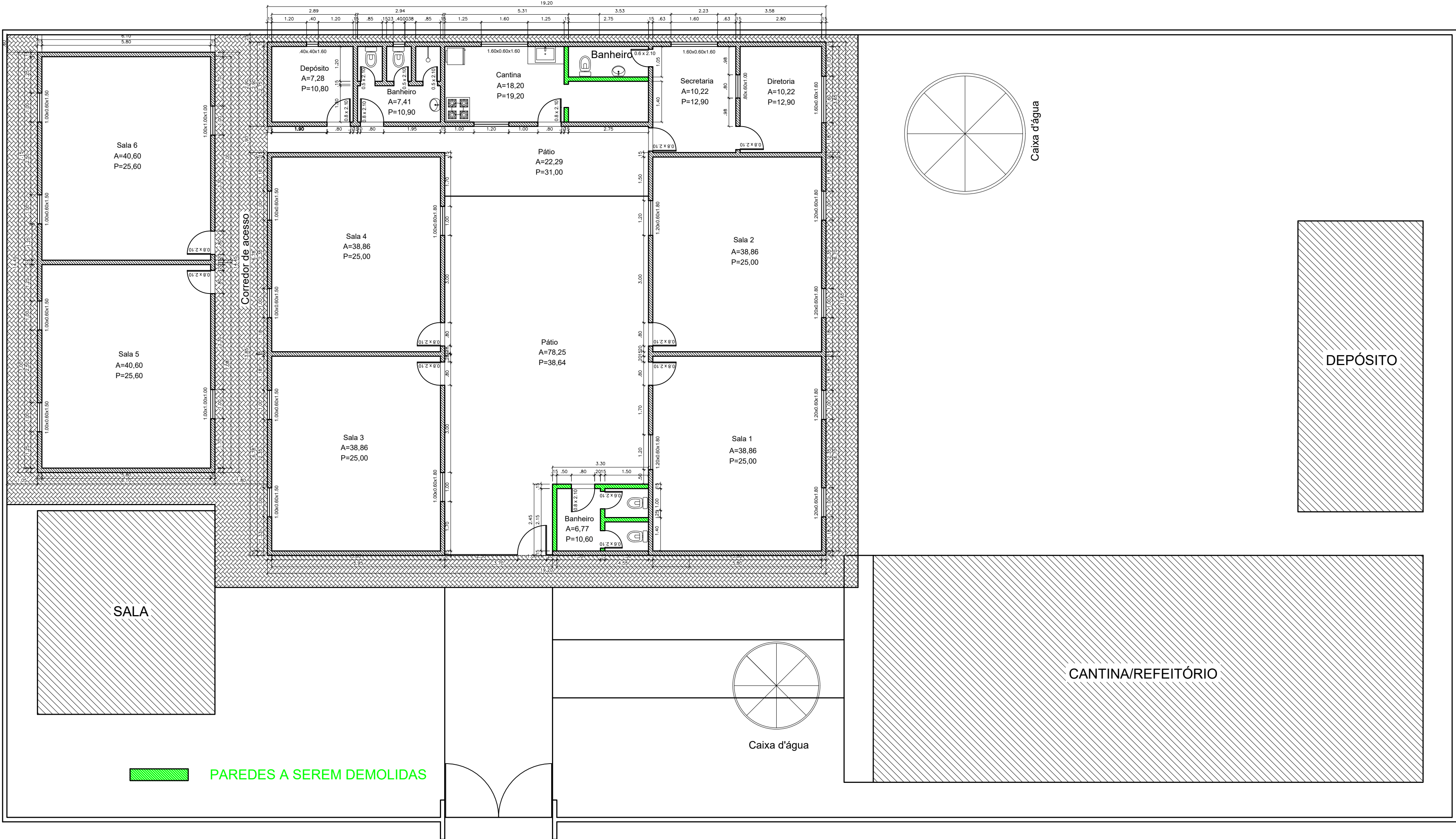
PLANTA BAIXA esc 1:100
