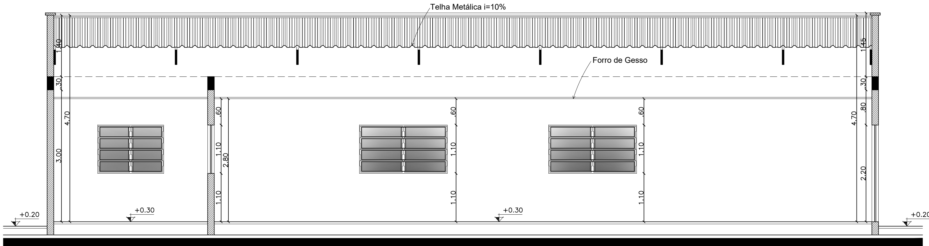
CORTE AA esc. 1:50
