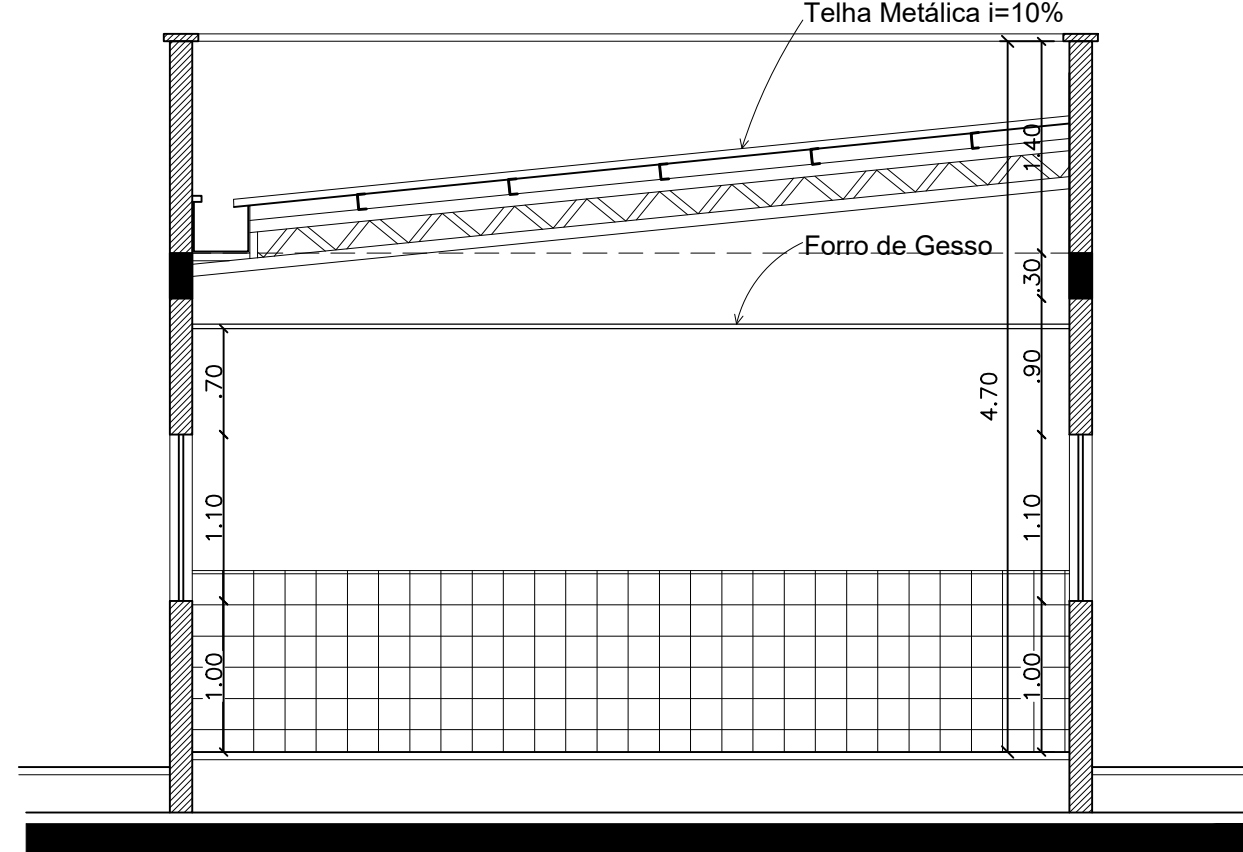
CORTE AA esc 1:75
