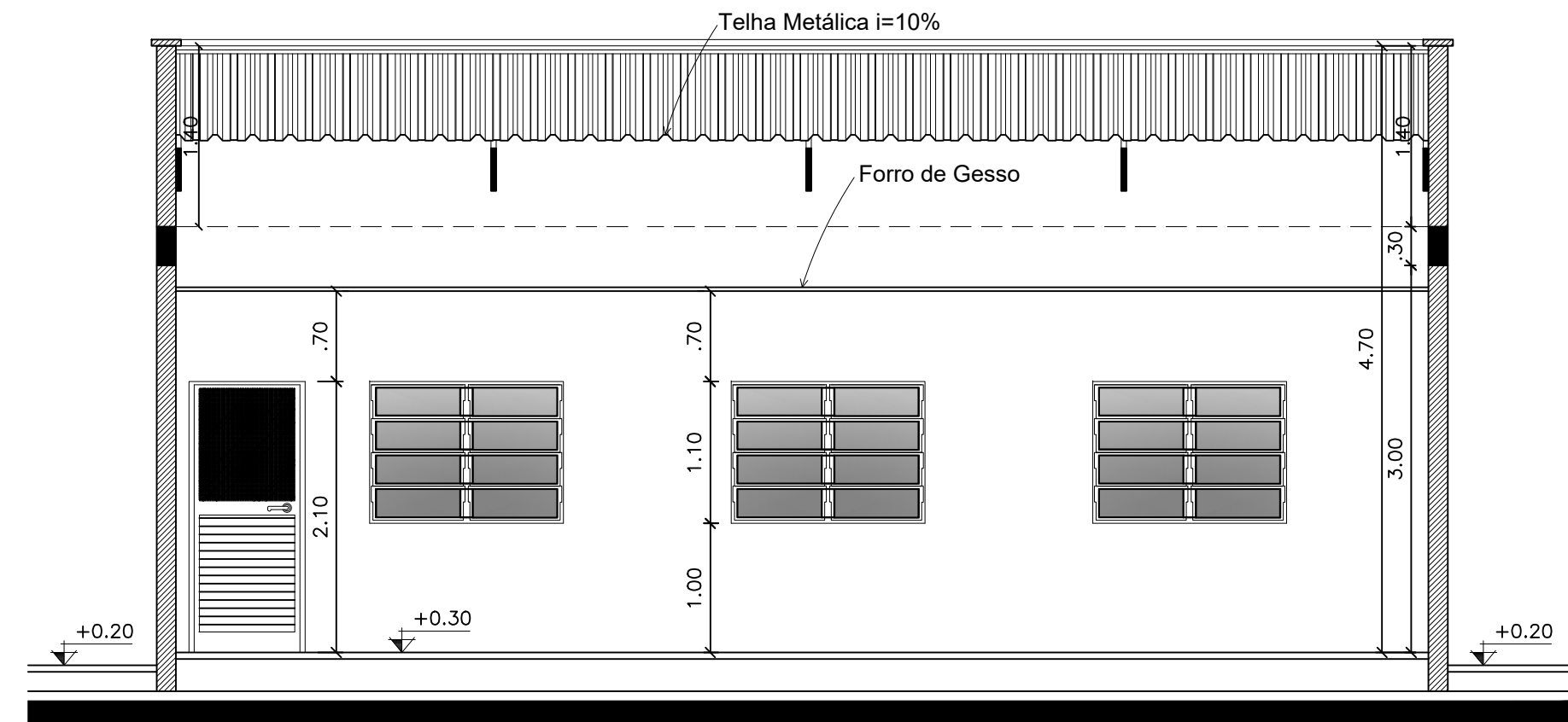
CORTE AA
