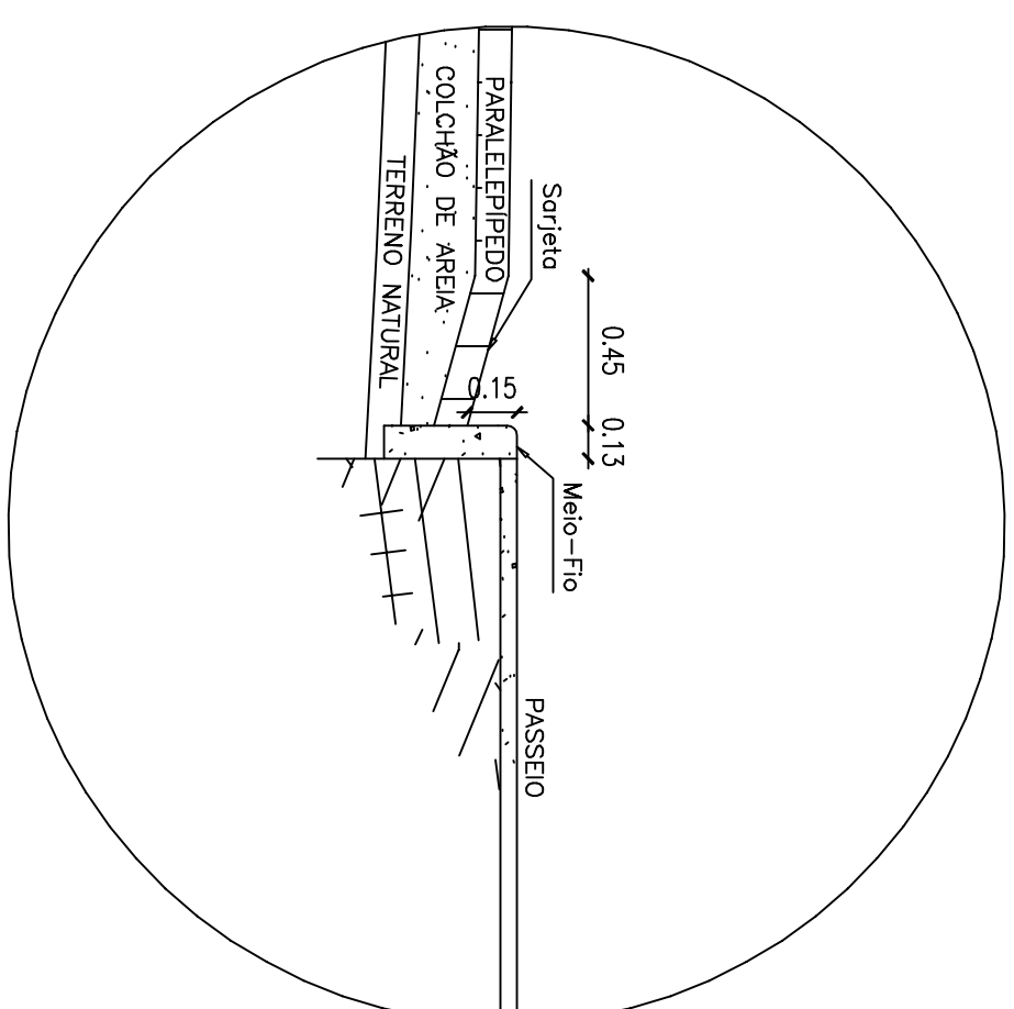
5 Detalhe da Sarjeta
