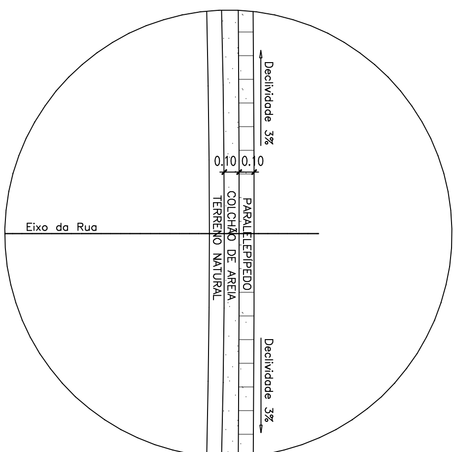
4 Detalhe Pavimentação
