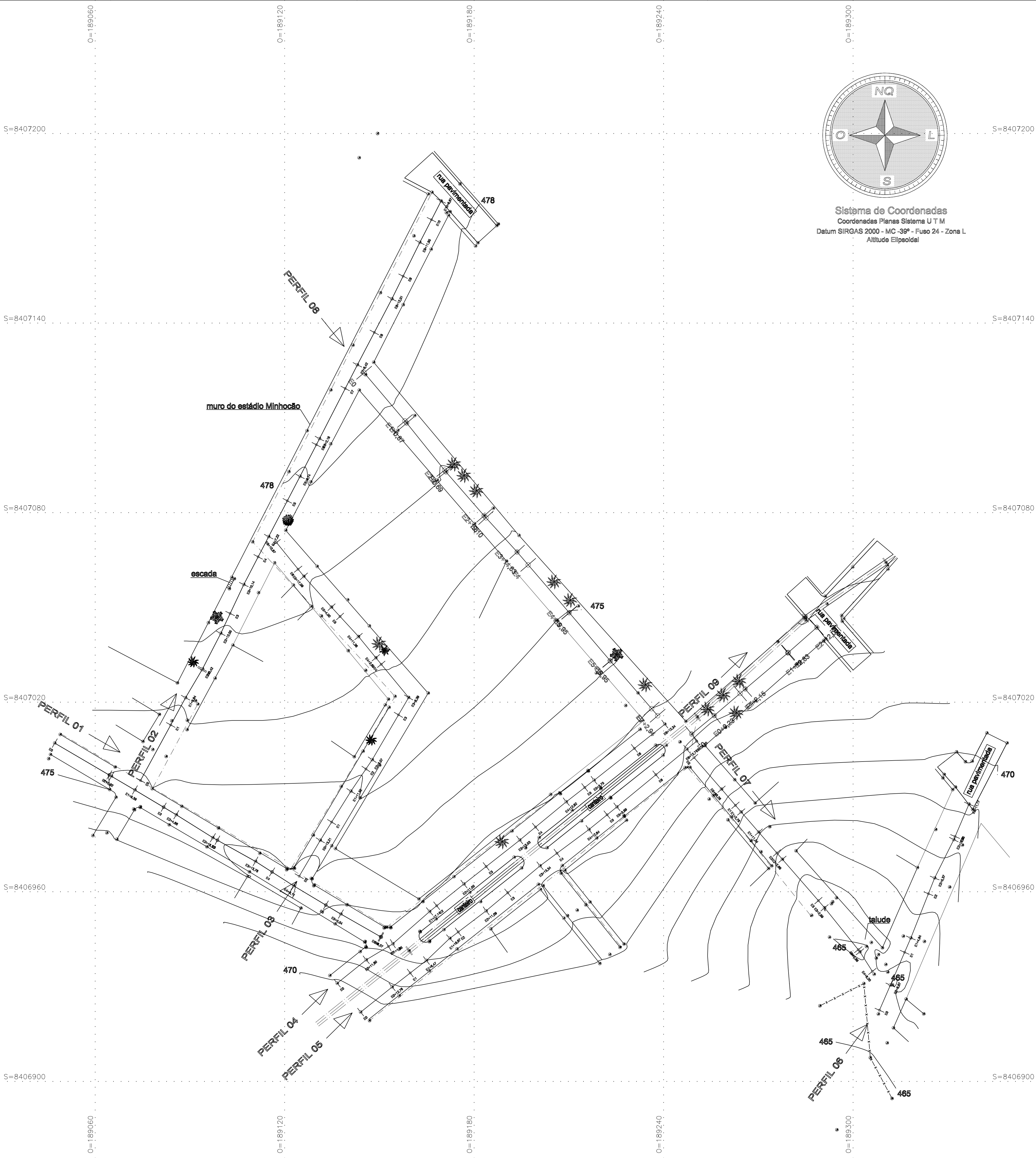
1 Planta de Levantamento Planialtimétrico ESCALA 1:600
