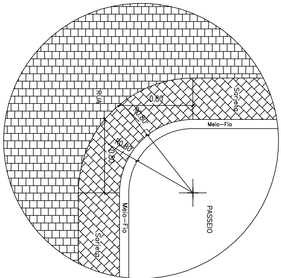
3 Detalhe da Curva ESCALA 1/25
