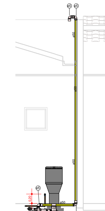
8 VISTA E 1 : 50
