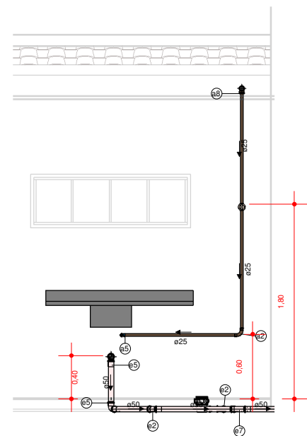
4 VISTA A 1 : 50
