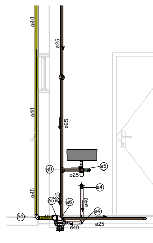
6 VISTA C 1 : 50
