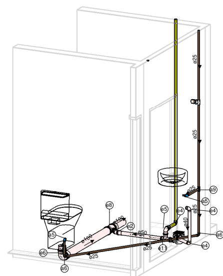
10 ISOMÉTRICO WC 01
