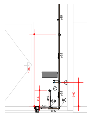
7 VISTA D 1 : 50
