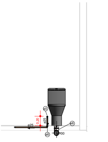
5 VISTA B 1 : 50
