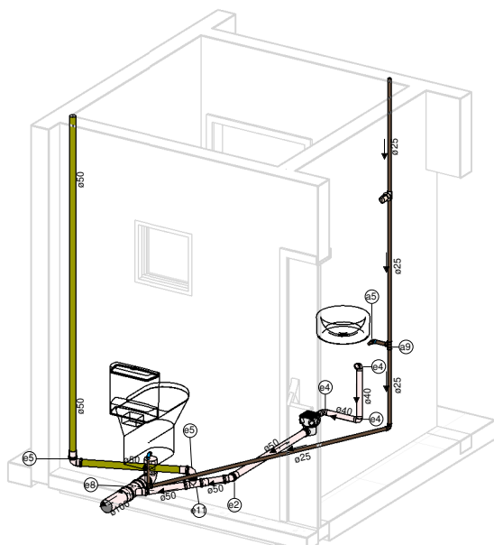
11 ISOMÉTRICO WC 02
