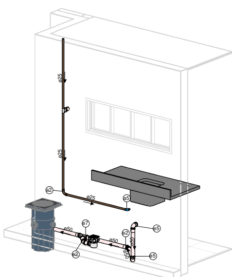
9 ISOMÉTRICO COZINHA
