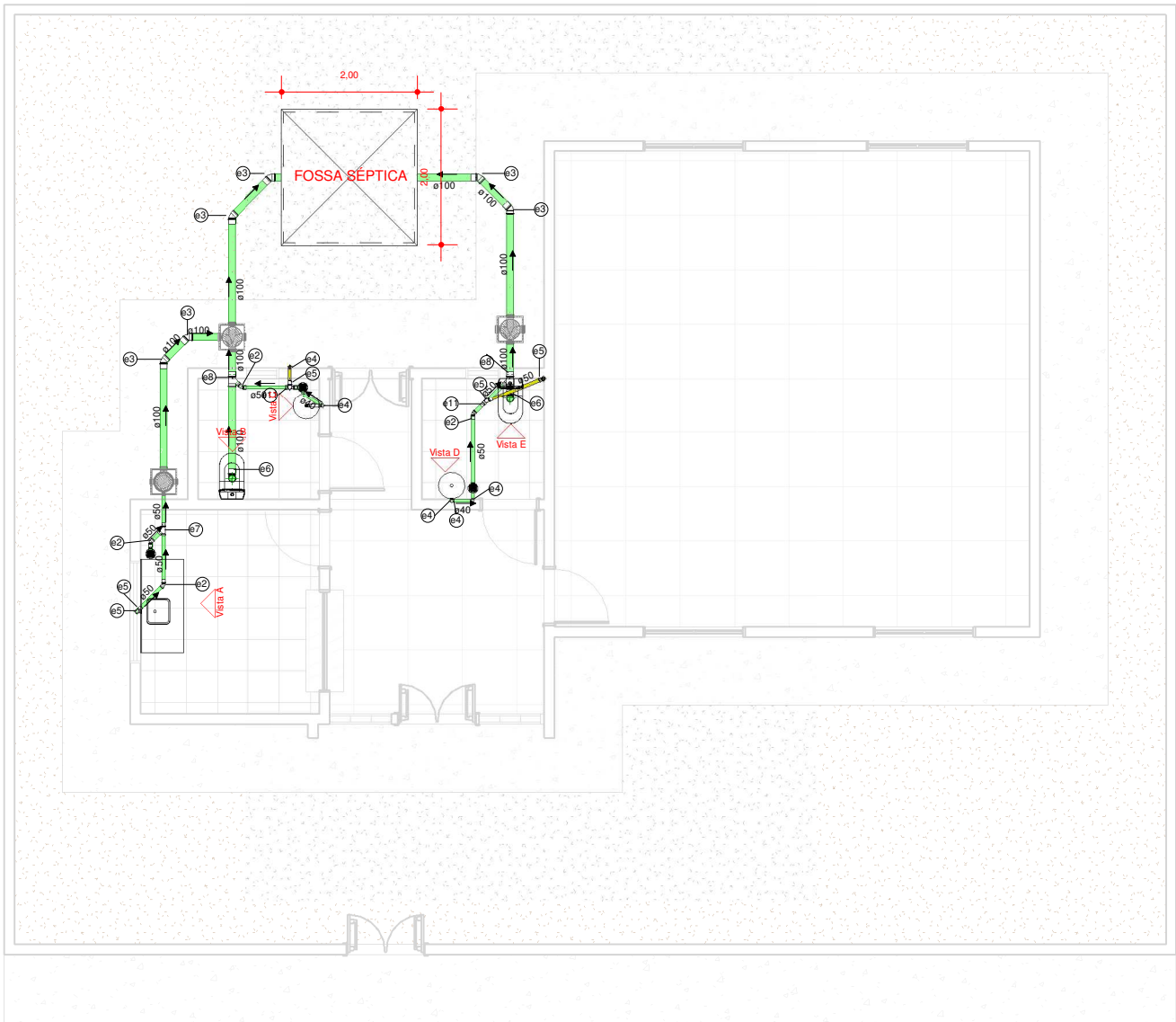
3 PLANTA DE ESGOTO 1 : 100
