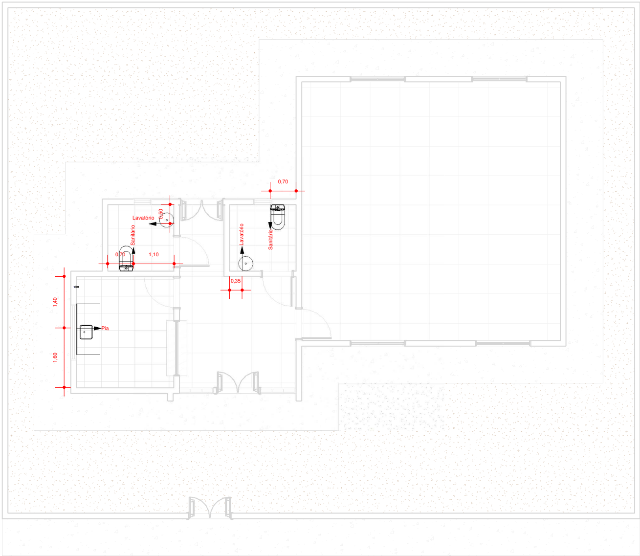
1 PLANTA DE PONTOS 1 : 100
