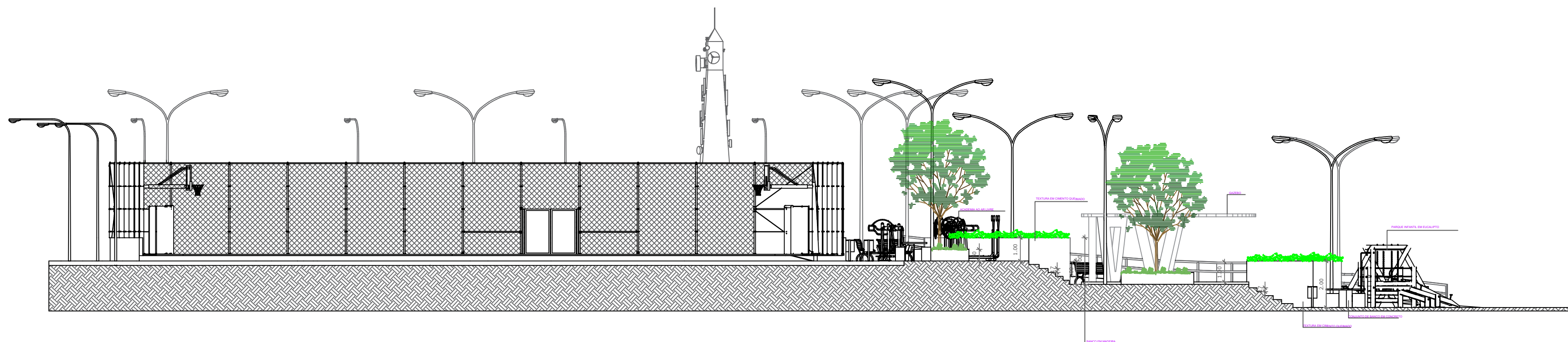
CORTE AA PRAÇA DO HOSPITAL
