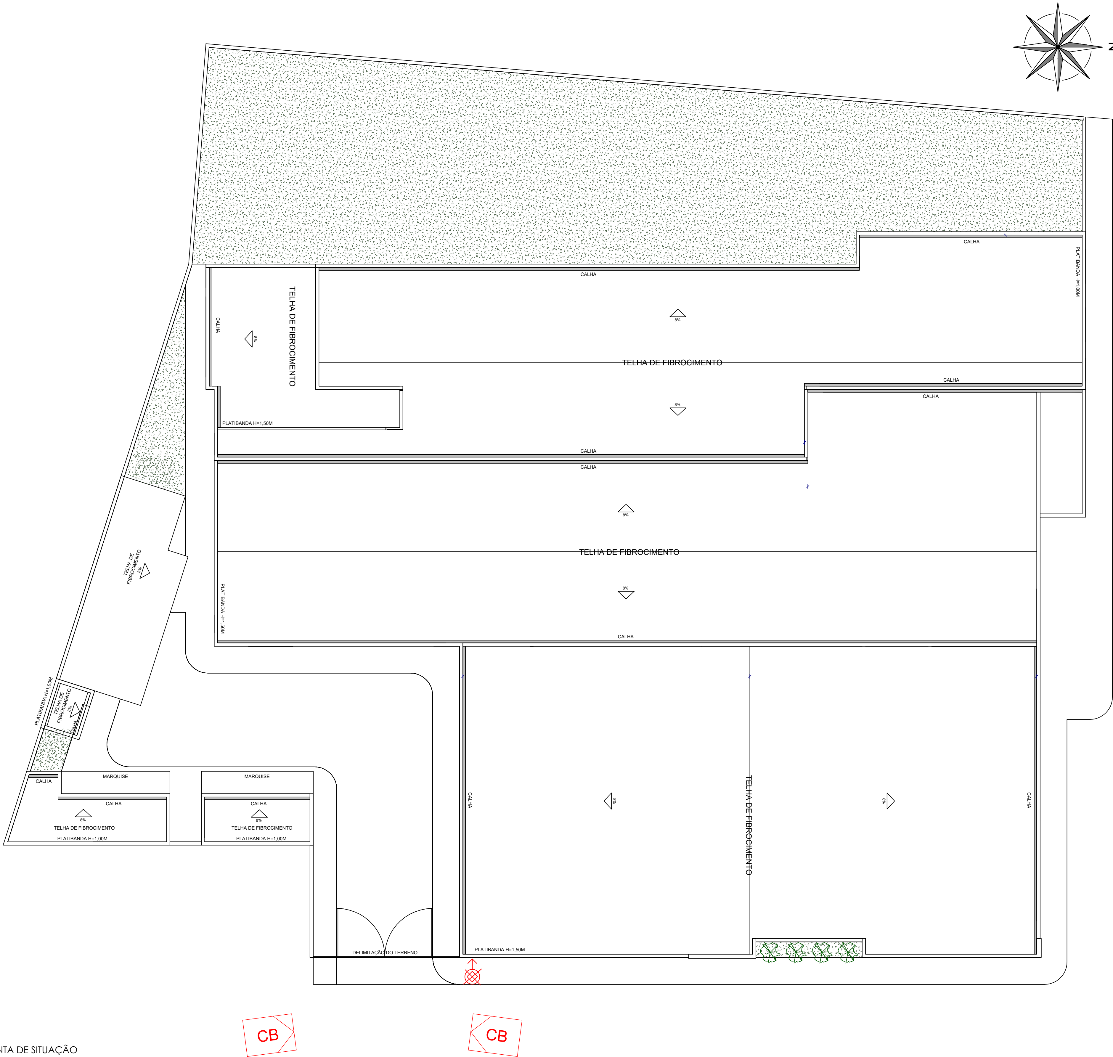
PLANTA DE SITUAÇÃO ESCALA 1/100 ÁREA CONSTRUÍDA TOTAL = 1080,07 m²
