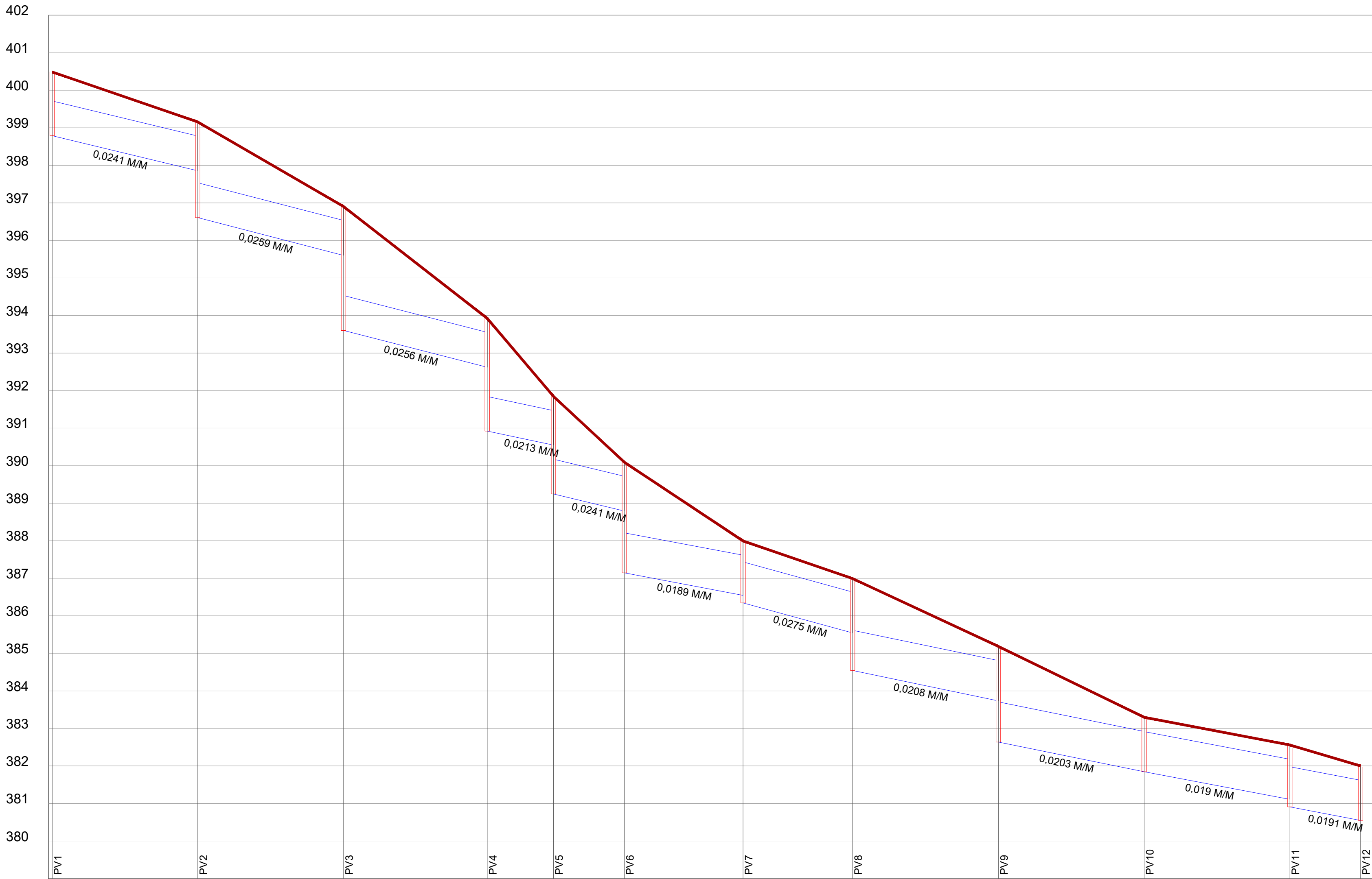
PERFIL DOS TRECHOS: PV1 AO PV12 ESCALA HORIZONTAL: 1:1000 ESCALA VERTICAL: 1:100
