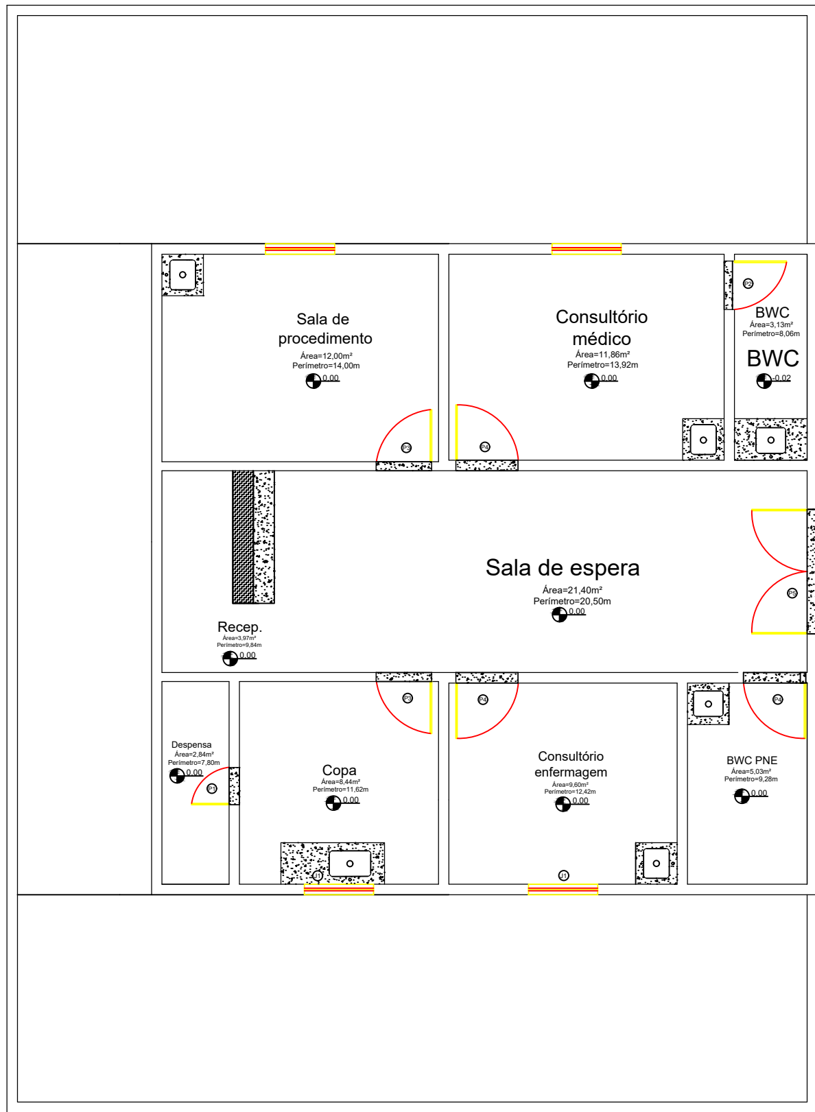
PLANTA DE SITUAÇÃO Esc:1/75
