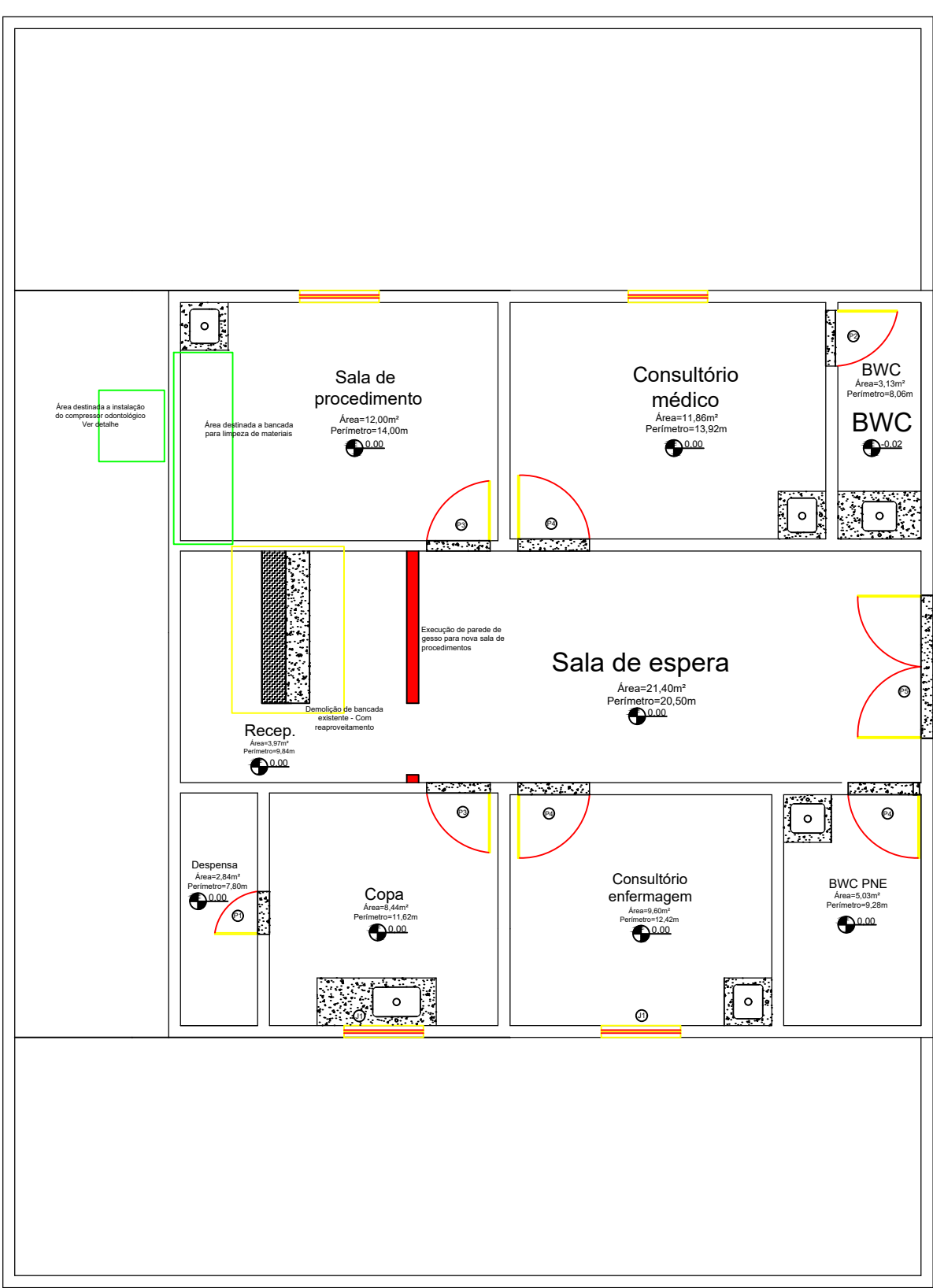
PLANTA DE REFORMA Esc:1/75
