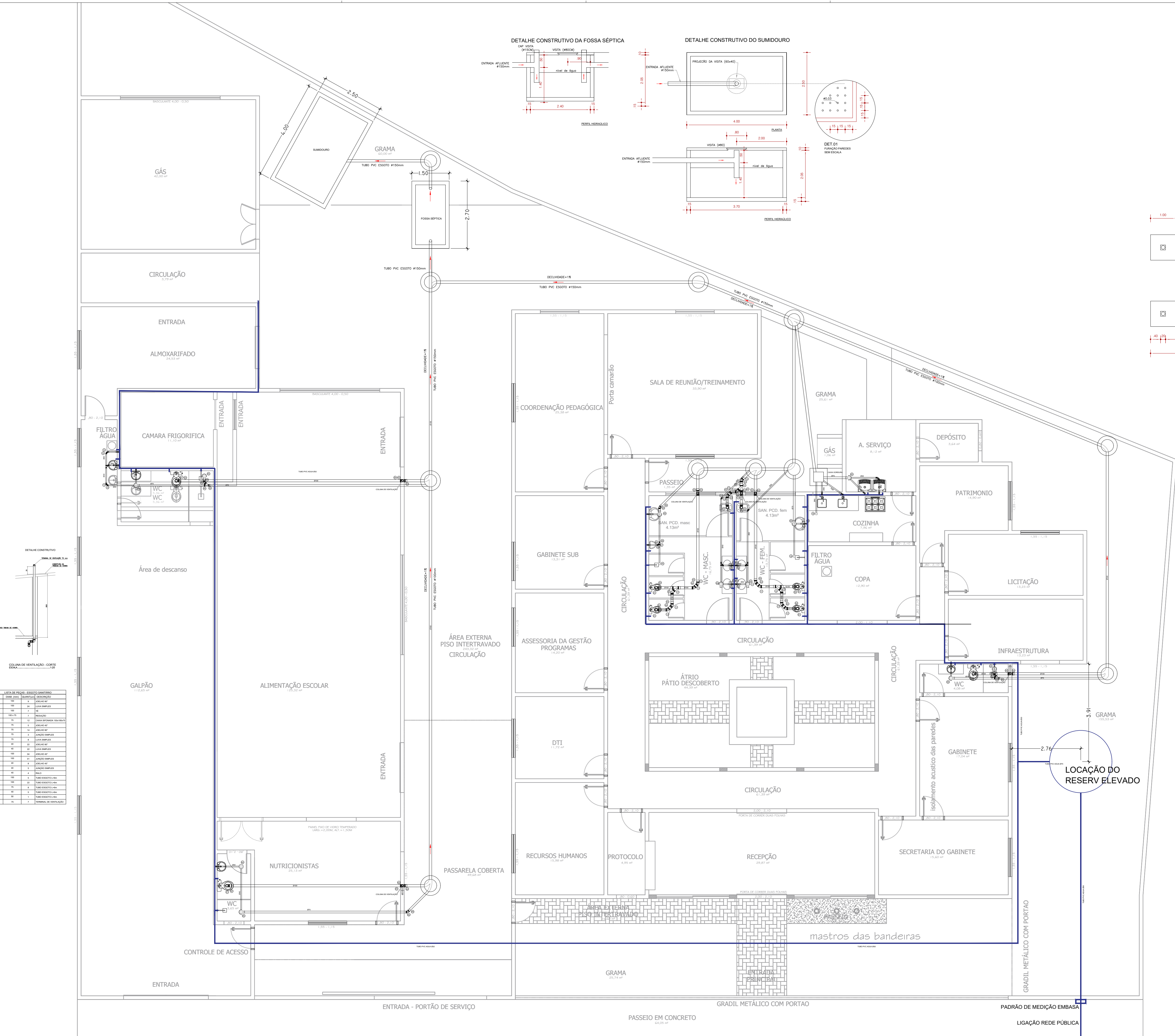
PLANTA BAIXA - HIDROSANITÁRIO SEDE SECRETARIA DE EDUCAÇÃO ESC.: 1/75
