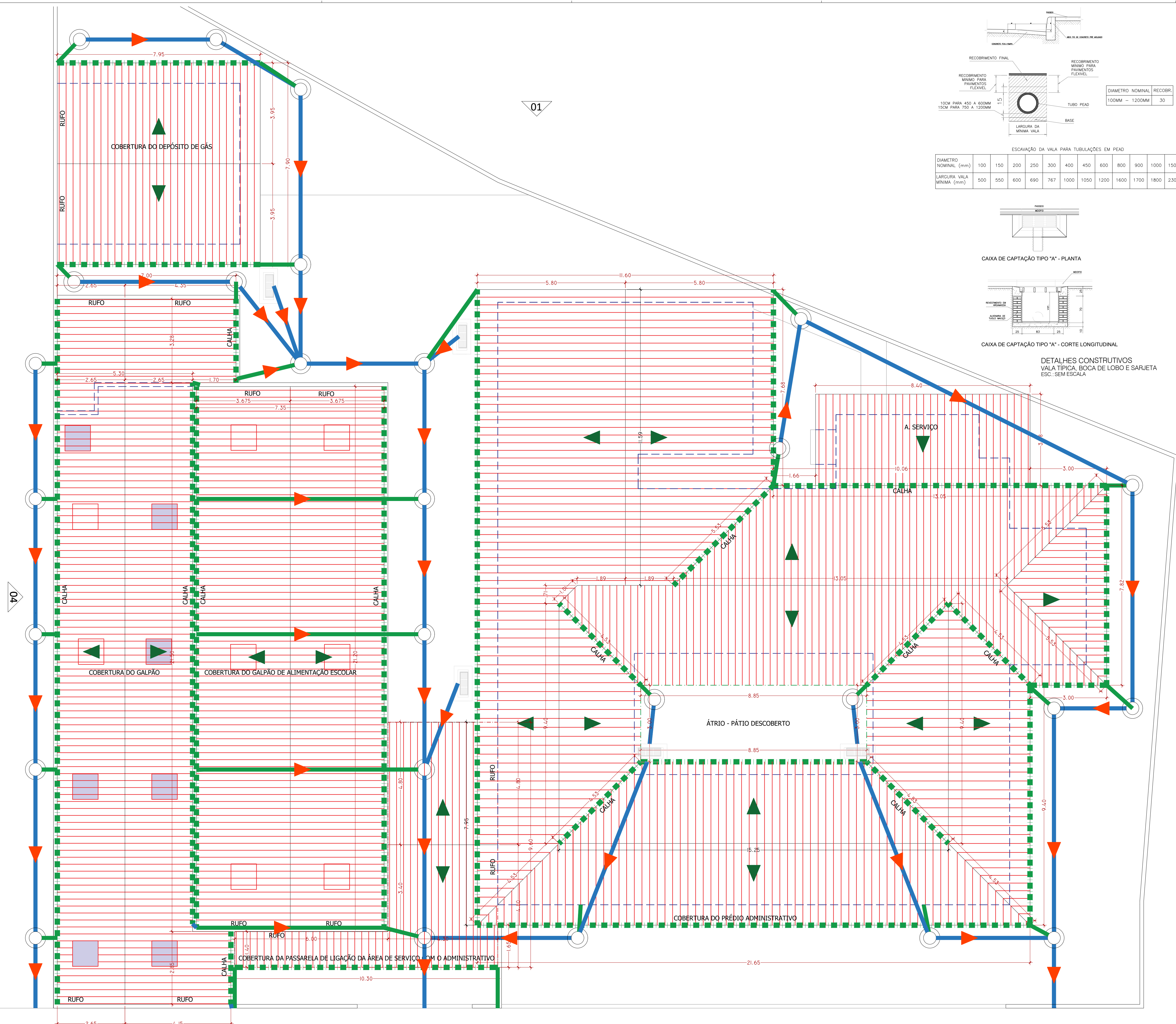
PLANTA BAIXA - DRENAGEM PLUVIAL SEDE SECRETARIA DE EDUCAÇÃO ESC.: 1/75
