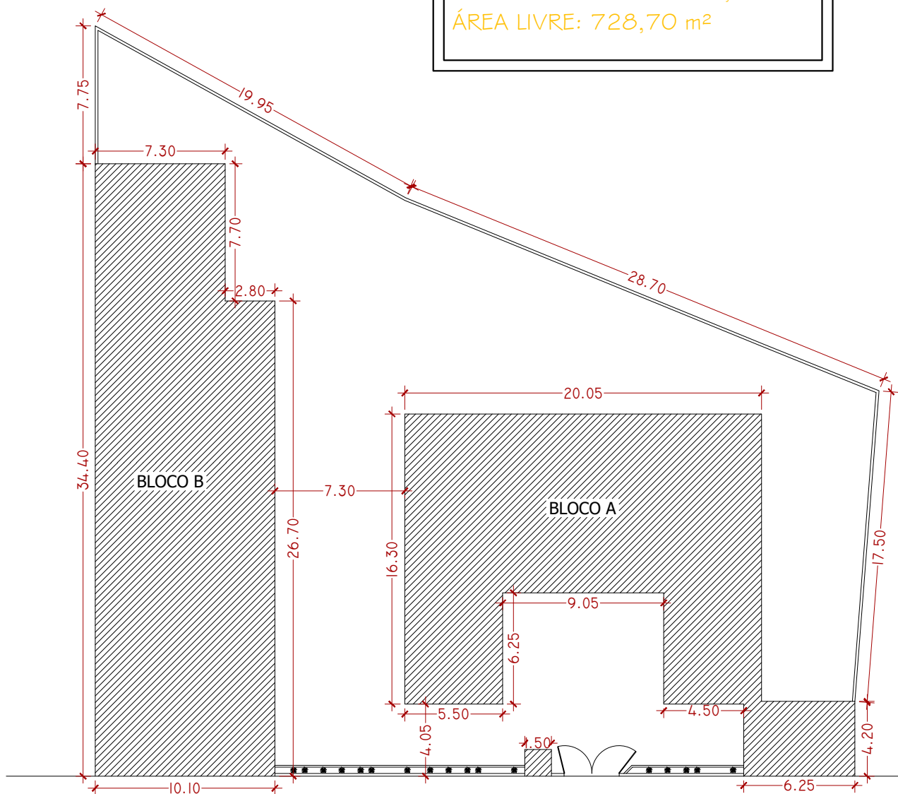
PLANTA DE SITUAÇÃO ESC 1:300
