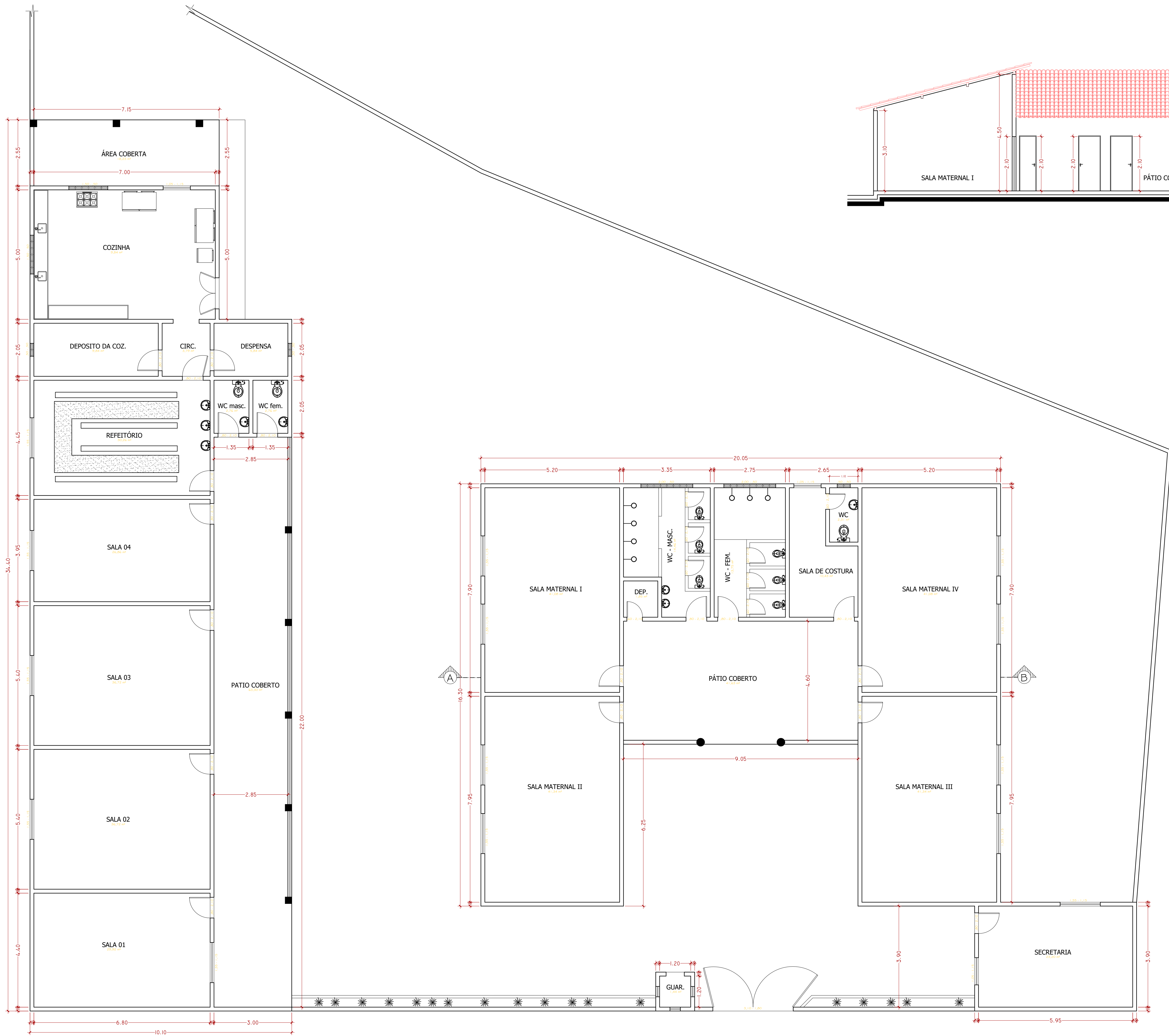
PLANTA BAIXA - CADASTRO SEDE SECRETARIA DE EDUCAÇÃO ESC.: 1/75
