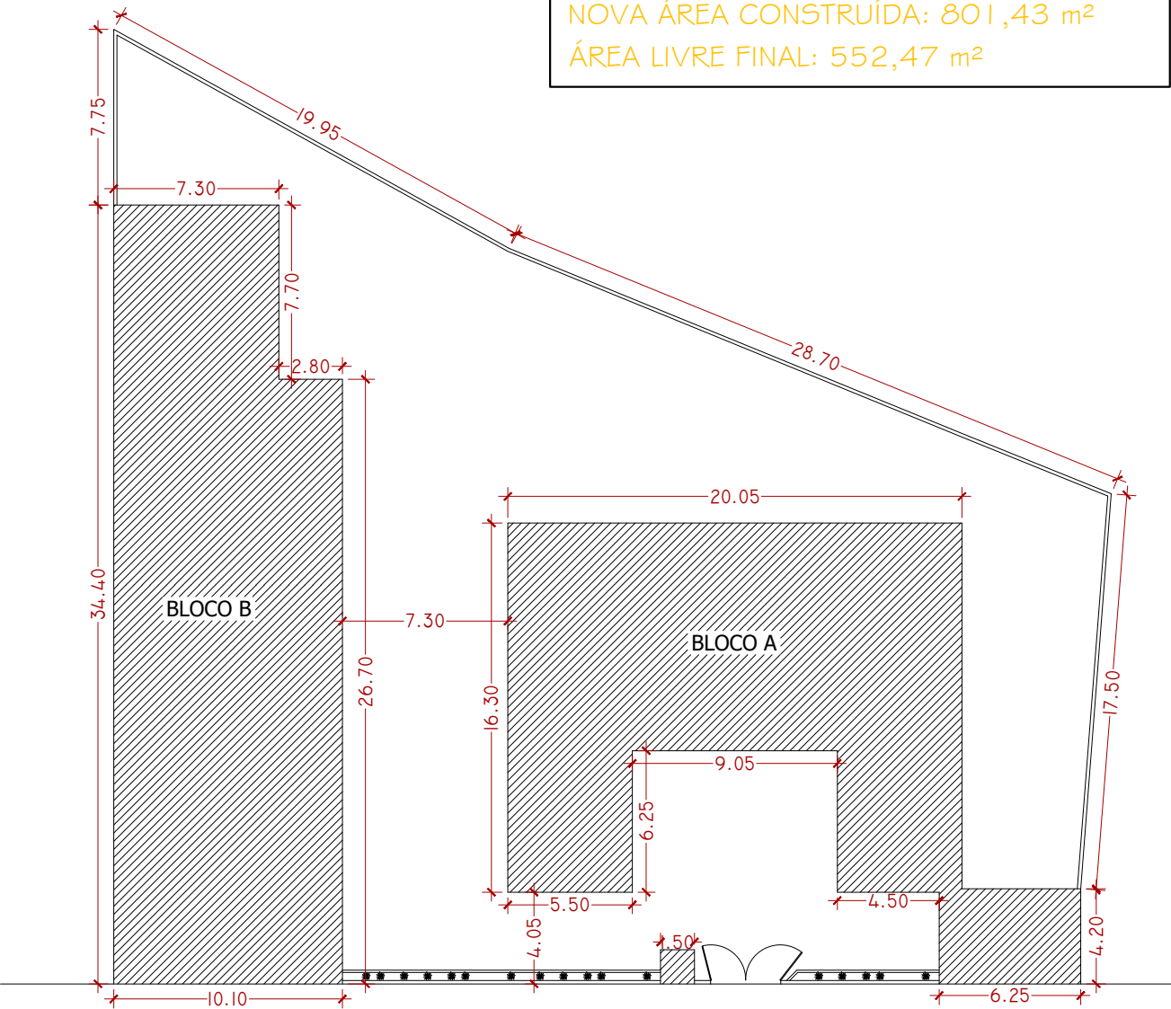
PLANTA DE SITUAÇÃO ESC 1:300
