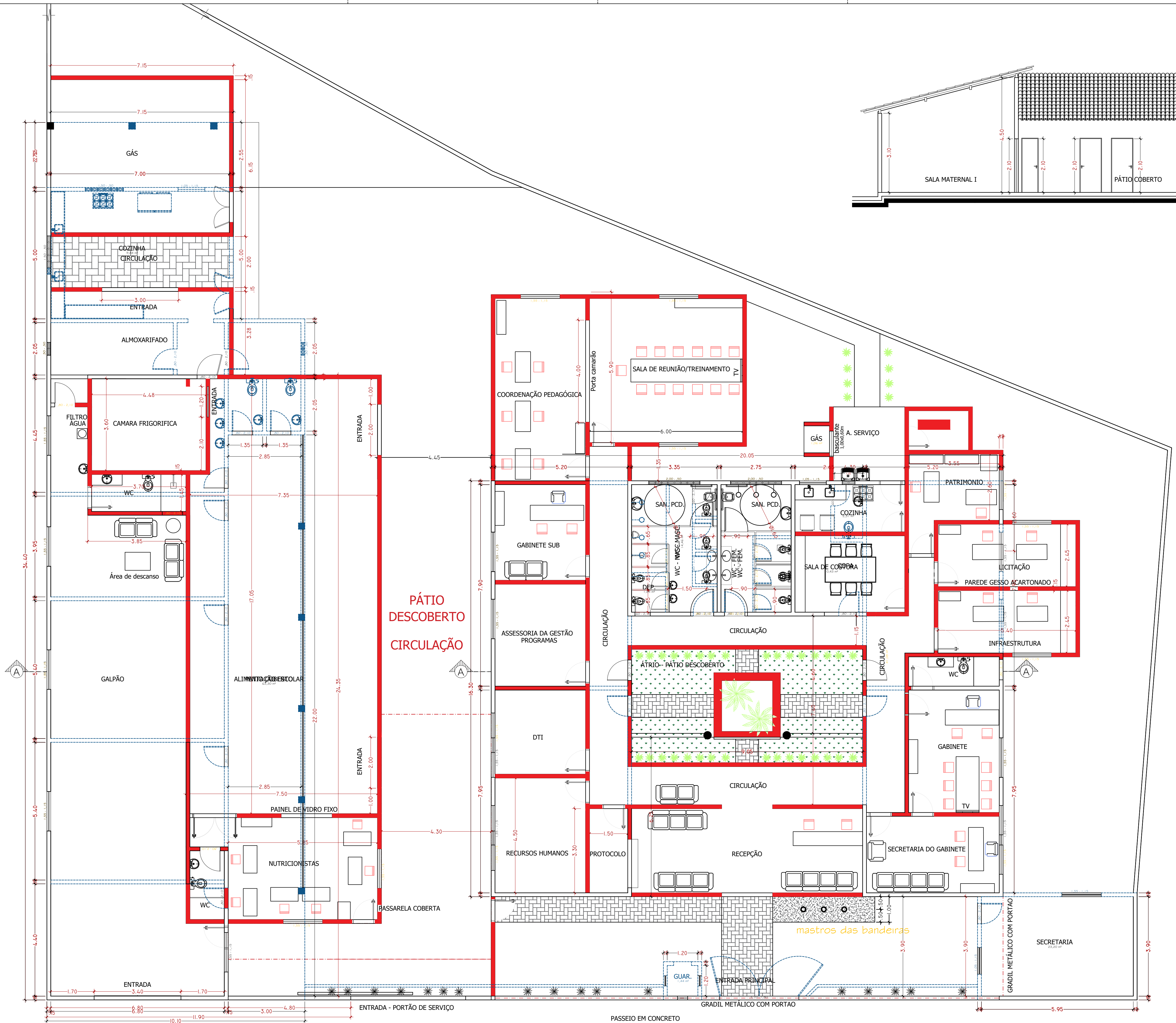
PLANTA CONSTRUÇÃO E DEMOLIÇÃO SEDE SECRETARIA DE EDUCAÇÃO ESC.: 1/75
