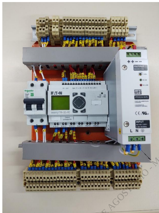
Figura 2: Exemplo de Painei de Automação
