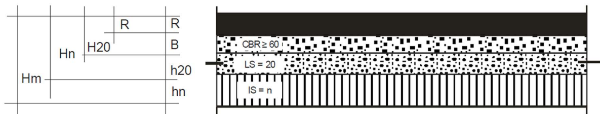
Dimensionamento do pavimento. Fonte: Manual de Pavimentação DNIT/2006.
