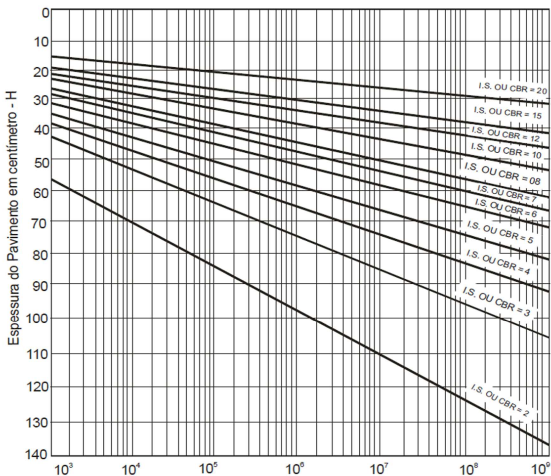
Ábaco de dimensionamento de pavimento flexível. Manual de Pavimentação DNIT/2006.
