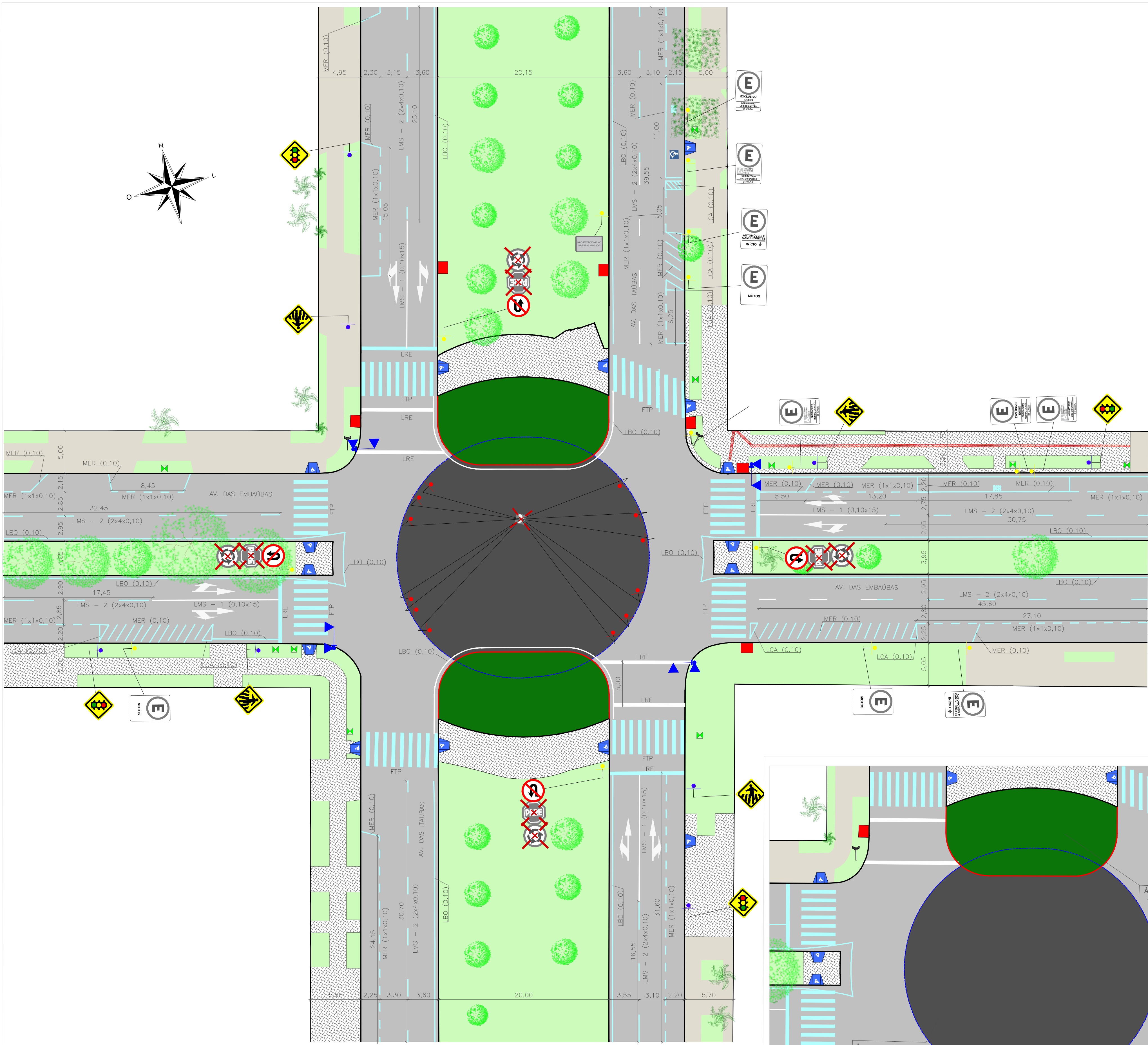
1 Implantação geral Escala 1:250
