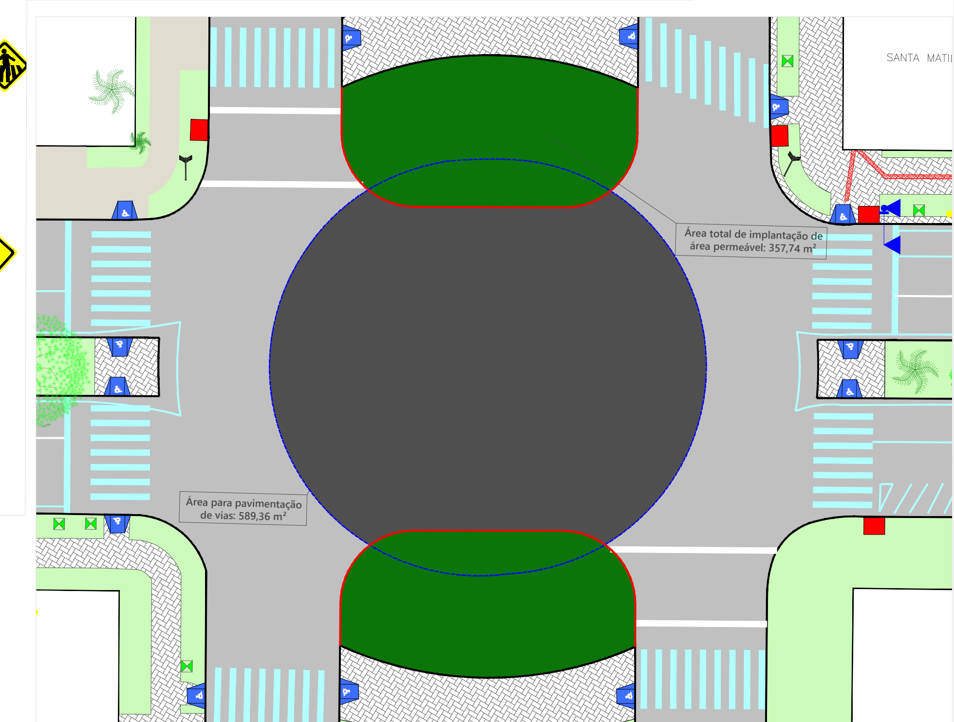
2 Detalhe pavimentação de calçadas e via Sem escala
