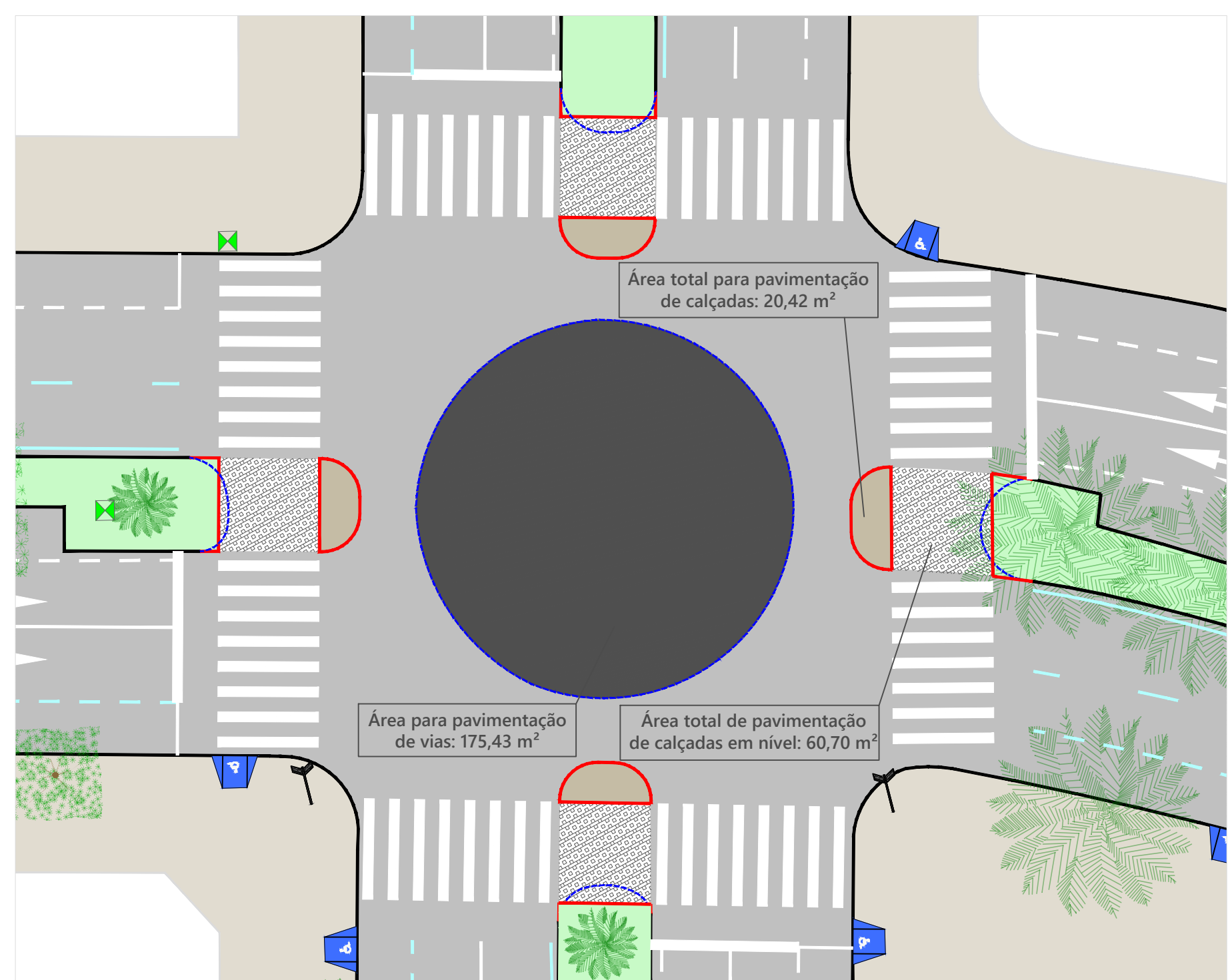
2 Detalhe pavimentação de calçadas e via Sem escala
