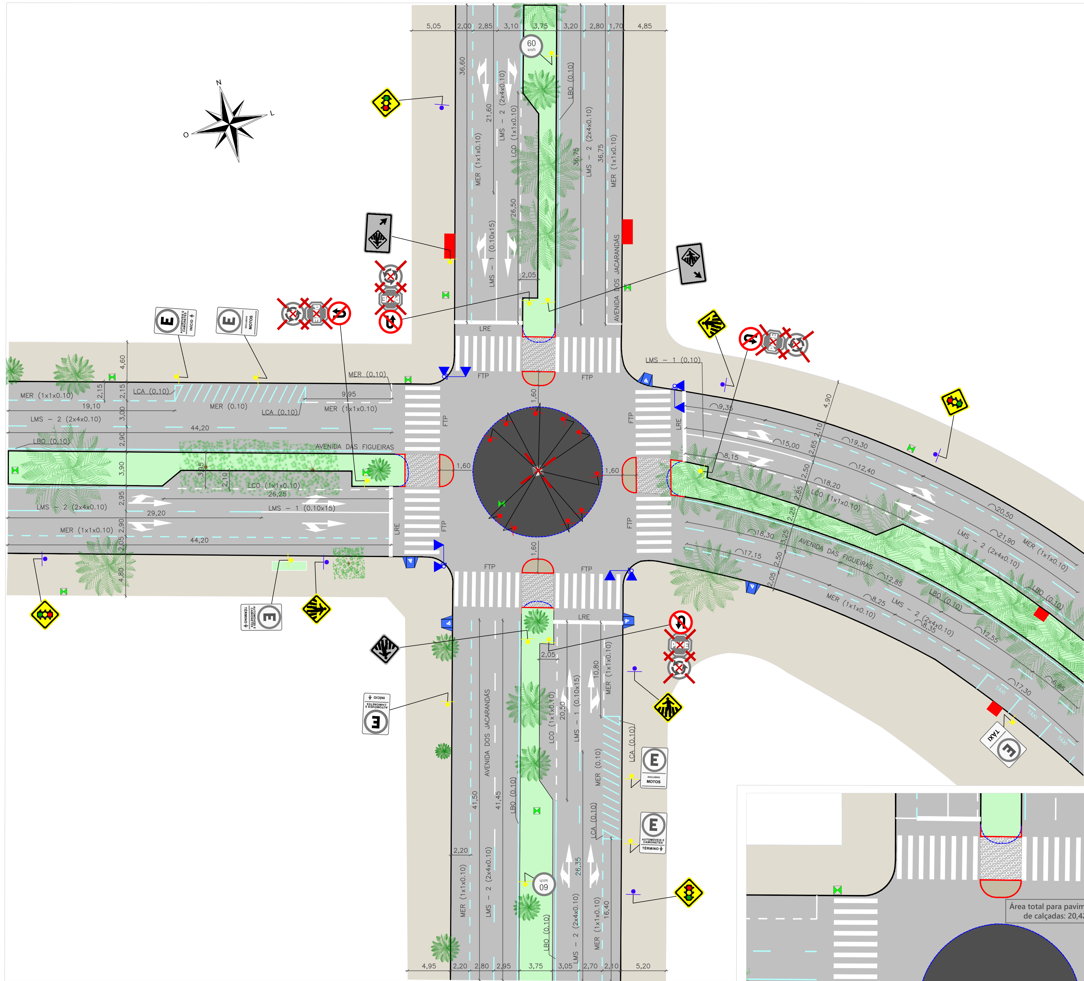
1 Implantação geral Escala 1:250
