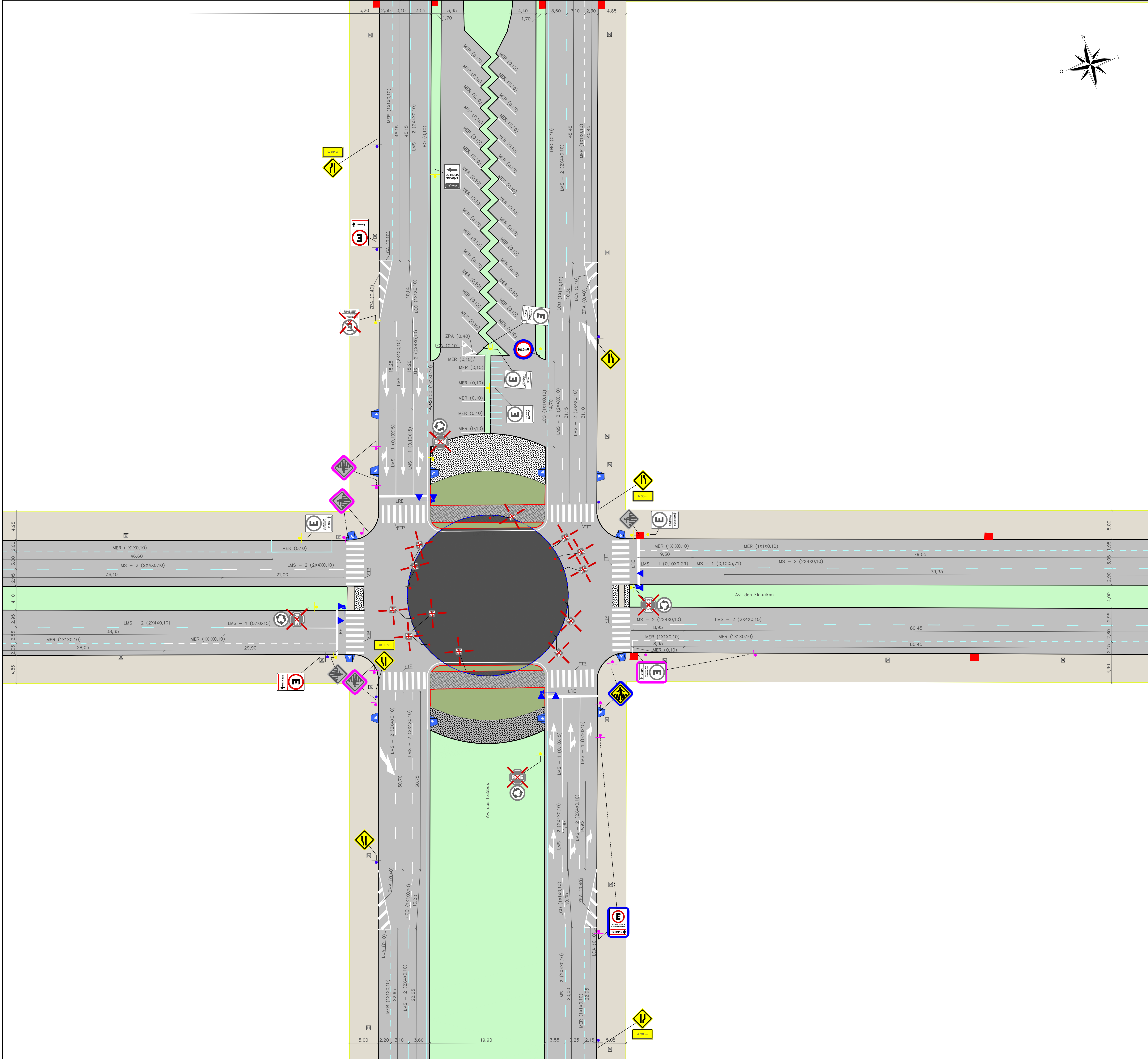
1 IMPLANTAÇÃO GERAL Escala: 1:250
