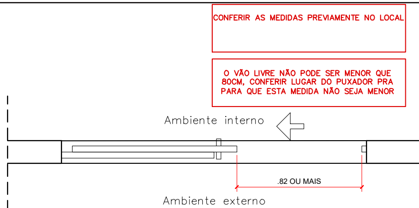
PLANTA PORTA ABERTA Escala 1/25
