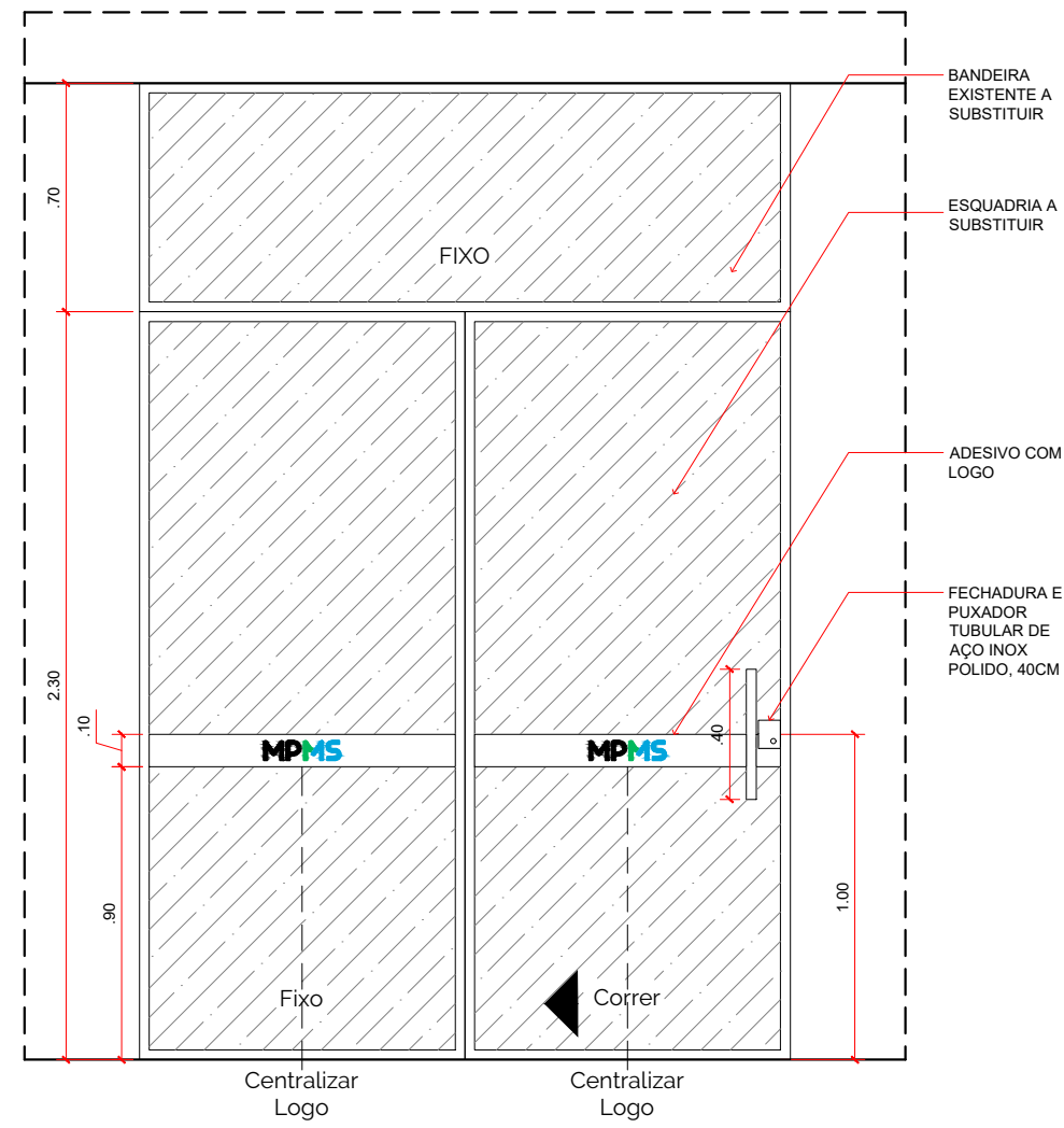
VISTA 1 PORTA DE VIDRO Escala 1/25
