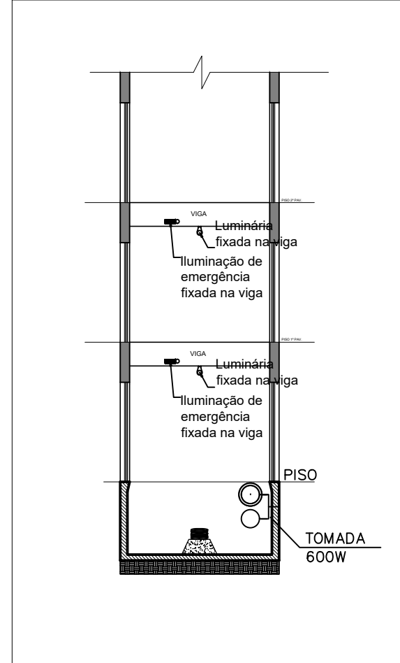
ILUMINAÇÃO - VIGA INTERMEDIÁRIA ESCALA 1:100
