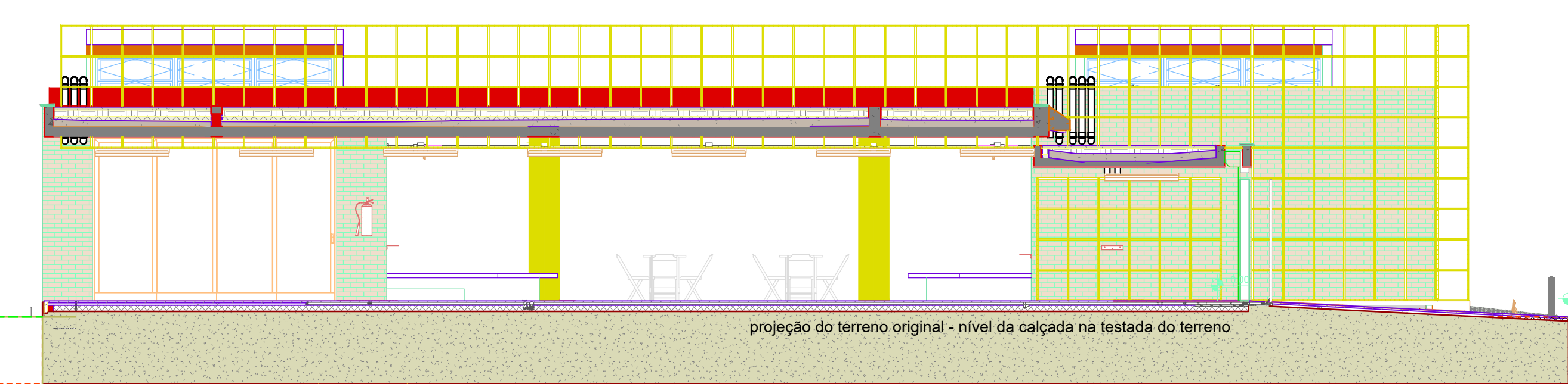
2 CORTE TERRENO 1:75
