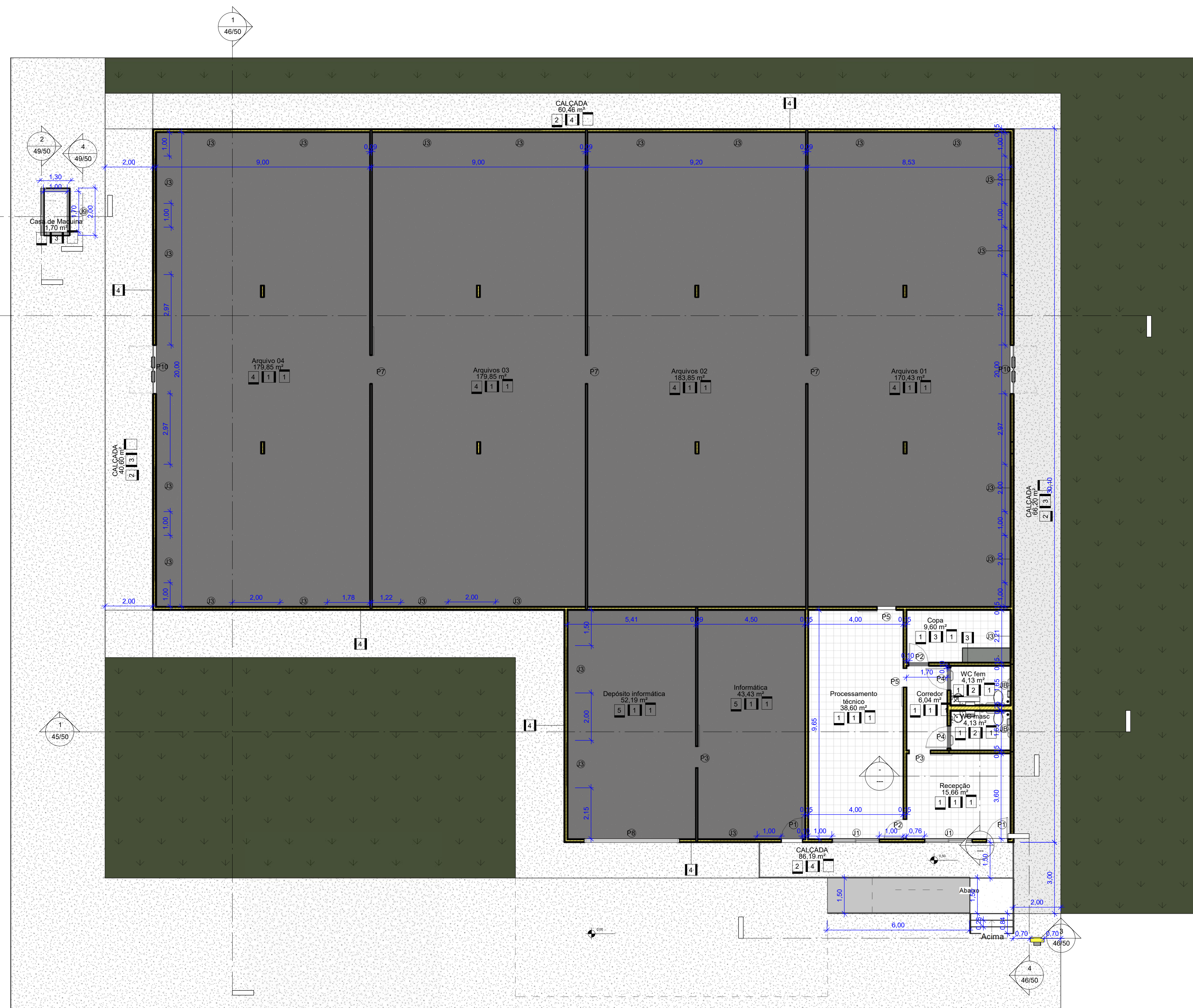
1 PLANTA BAIXA EXECUÇÃO escala 1 : 100
