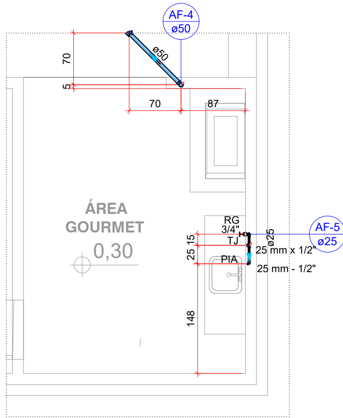
4 DETALHE 2 - ÁREA GOURMET - PLANTA BAIXA 1:50
