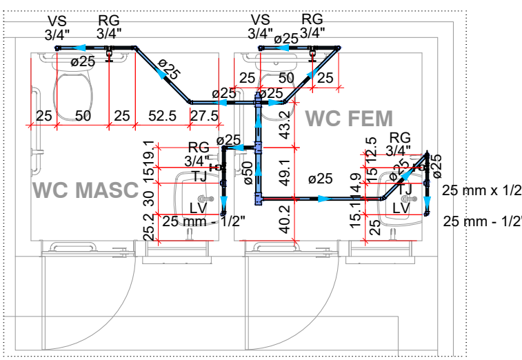
6 DETALHE 3 - BANHEIROS - PLANTA BAIXA 1:50
