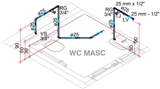
7 ISOMÉTRICO 3 - WC MASC - PLANTA BAIXA 1:500
