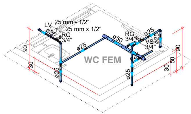
8 ISOMÉTRICO 4 - WC FEM - PLANTA BAIXA 1:50
