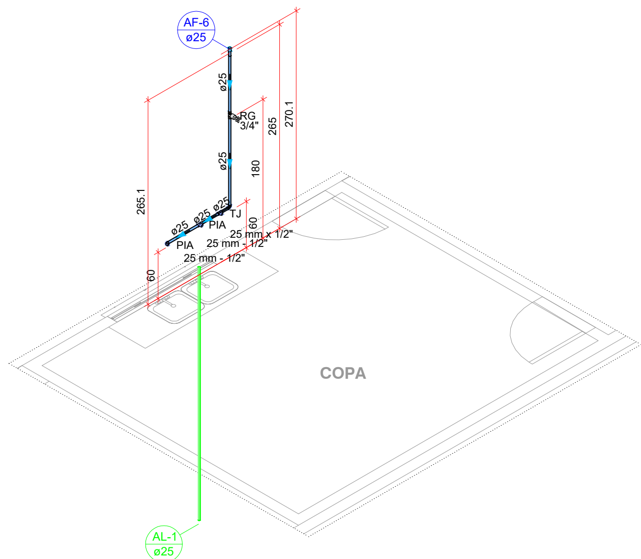
3 ISOMÉTRICO 1 - COPA - PLANTA BAIXA 1:50
