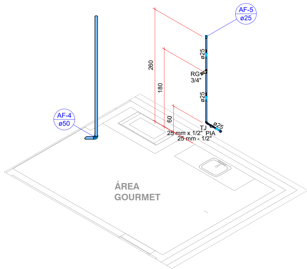
5 ISOMÉTRICO 2 - ÁREA GOURMET - PLANTA BAIXA 1:50
