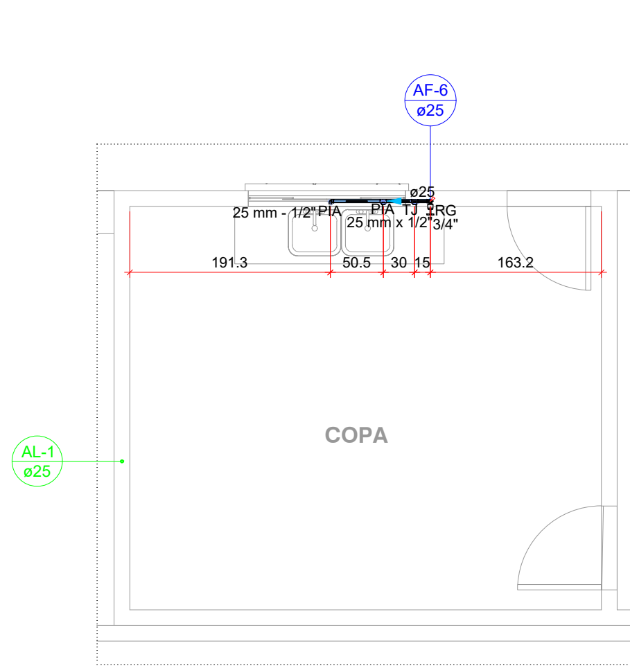
2 DETALHE 1 - COPA - PLANTA BAIXA 1:50
