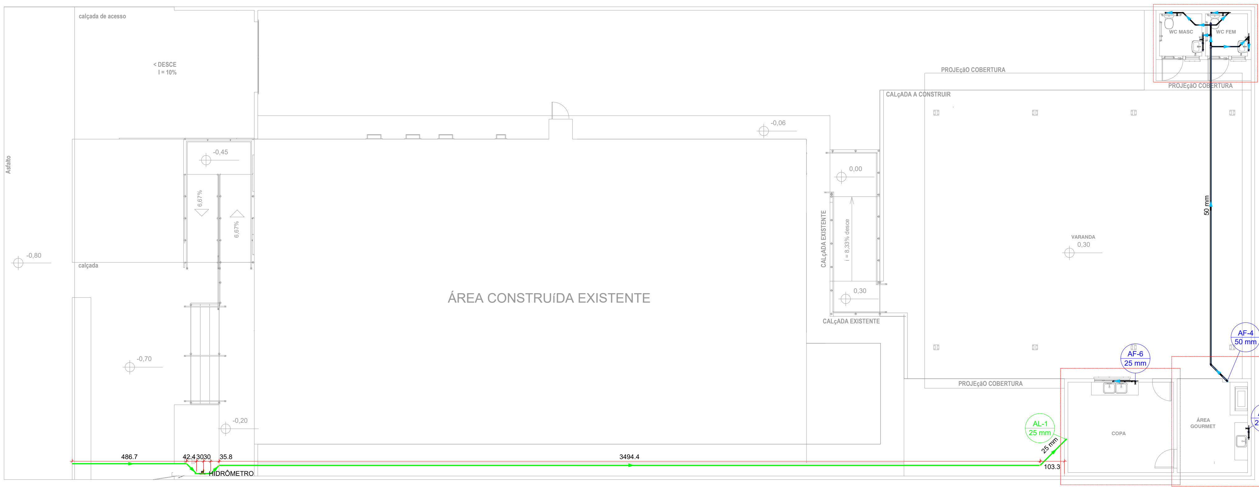
1 PLANTA BAIXA - HIDRAULICO 1:100
