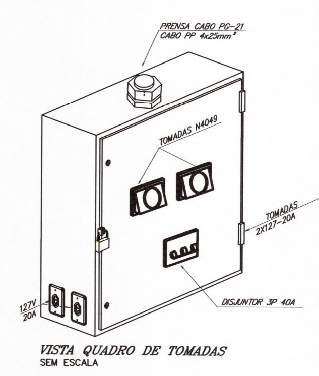
DET: CAIXA DE ATERRAMENTO SEM ESCALA
