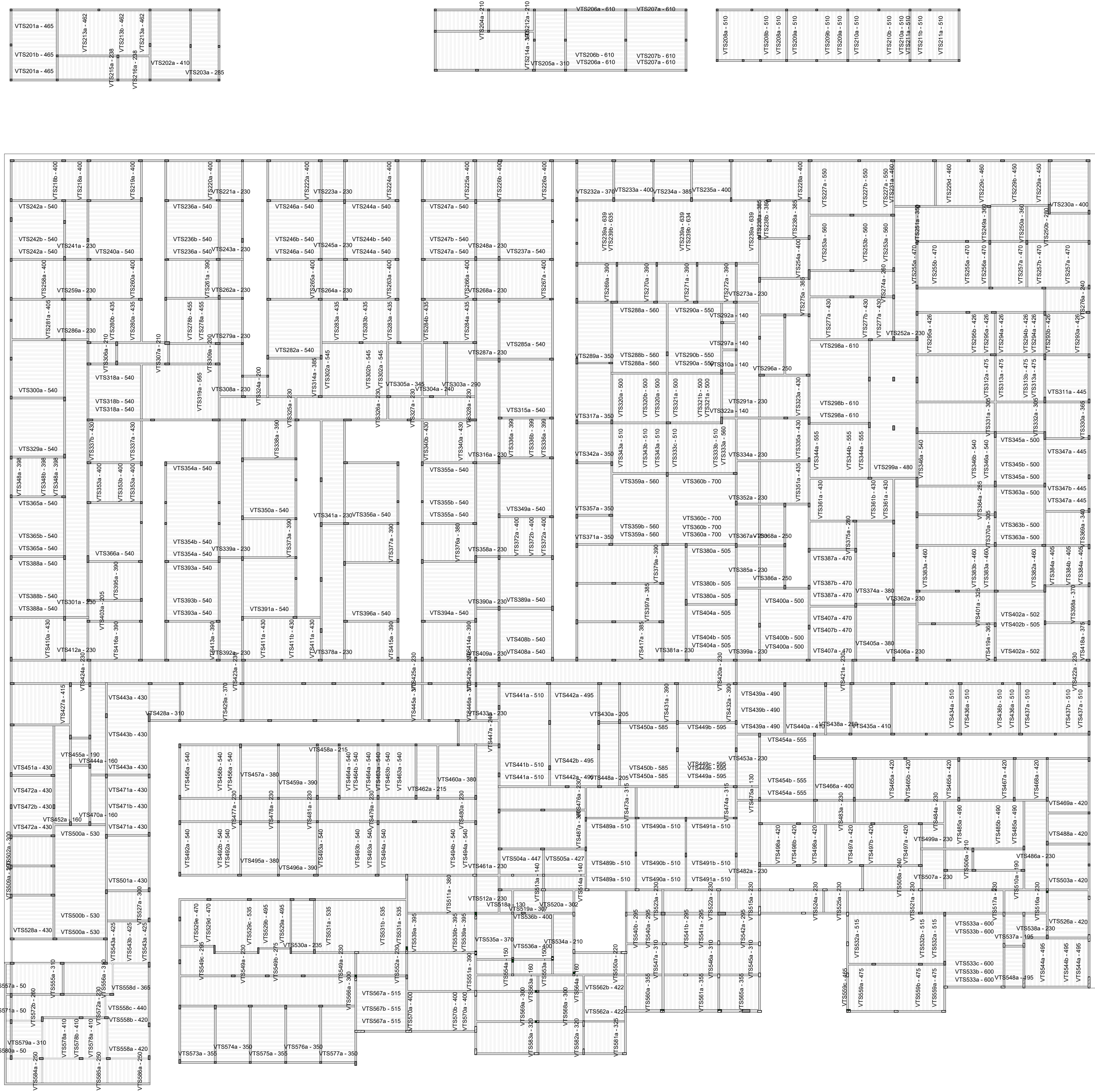
Planta de vigotas pré-moldadas escala 1:200
