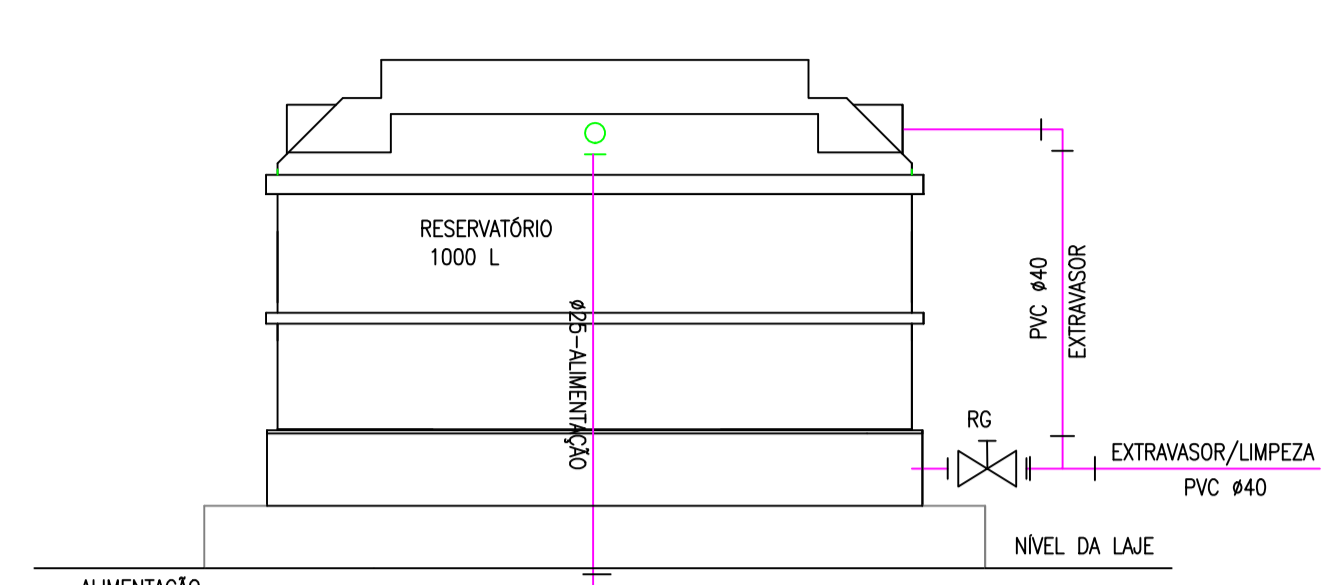
RESERVATÓRIO AF SOBRE A LAJE SEM ESCALA
