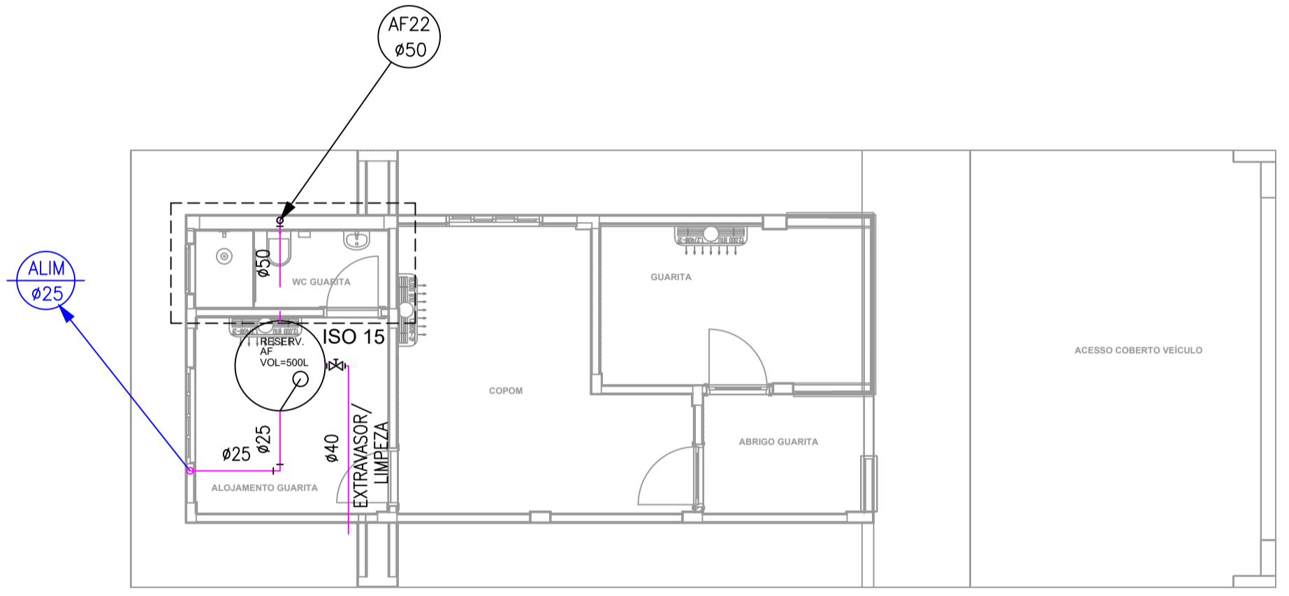
GUARITA ESCALA 1:75
