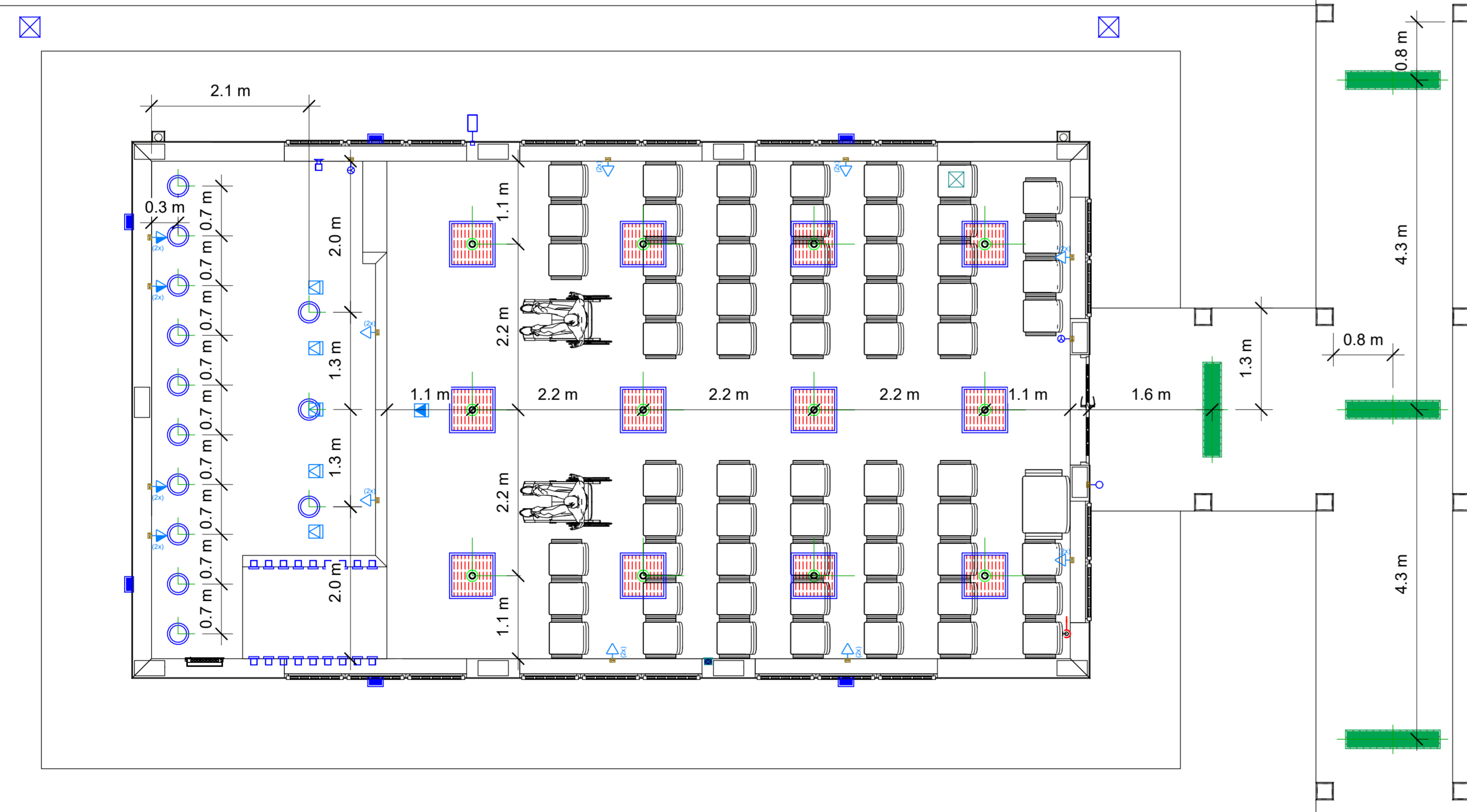
1 Locação de Pontos de Iluminação Blocos 2 e 3 1 : 50
