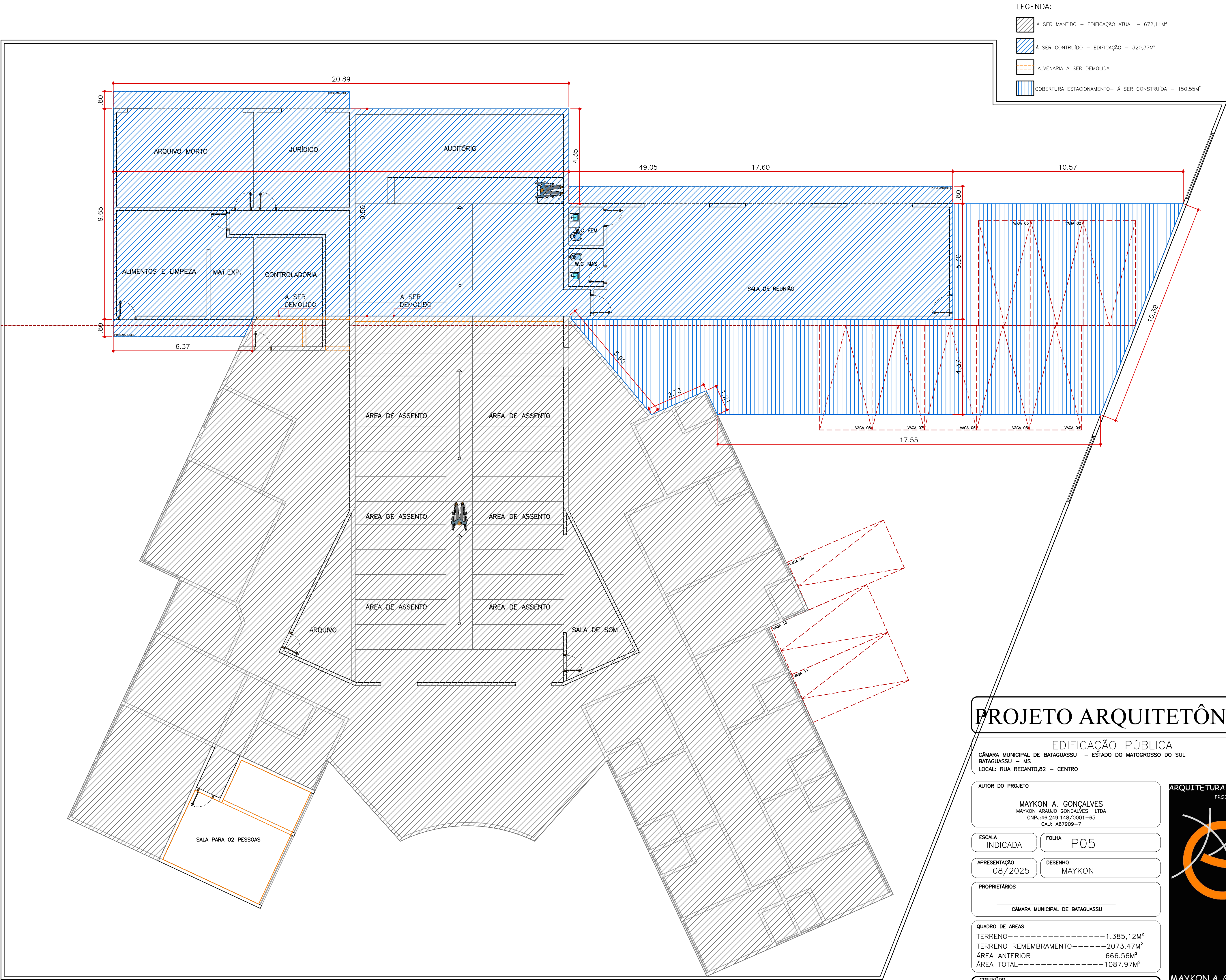
PLANTA BAIXA DEMOLIDO/CONSTRUÍDO ESC:1/100
