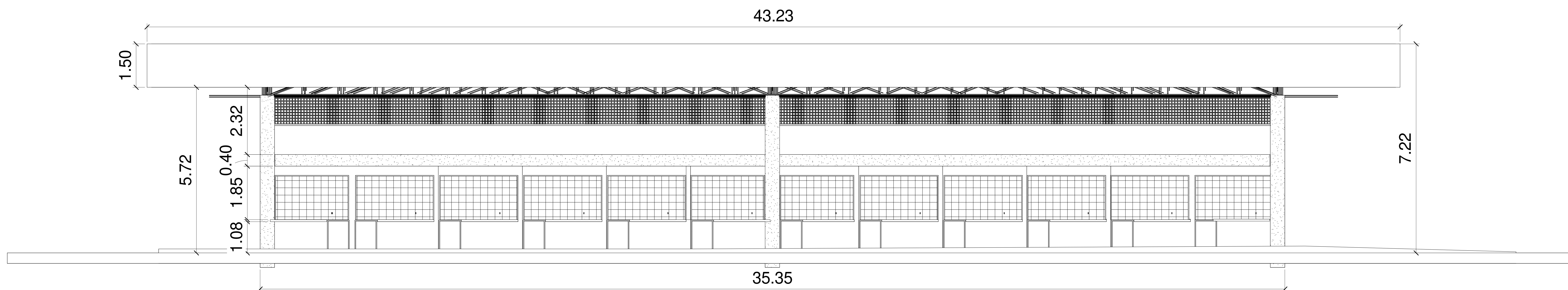
2 LATERAL ESQUERDA 1 : 50
