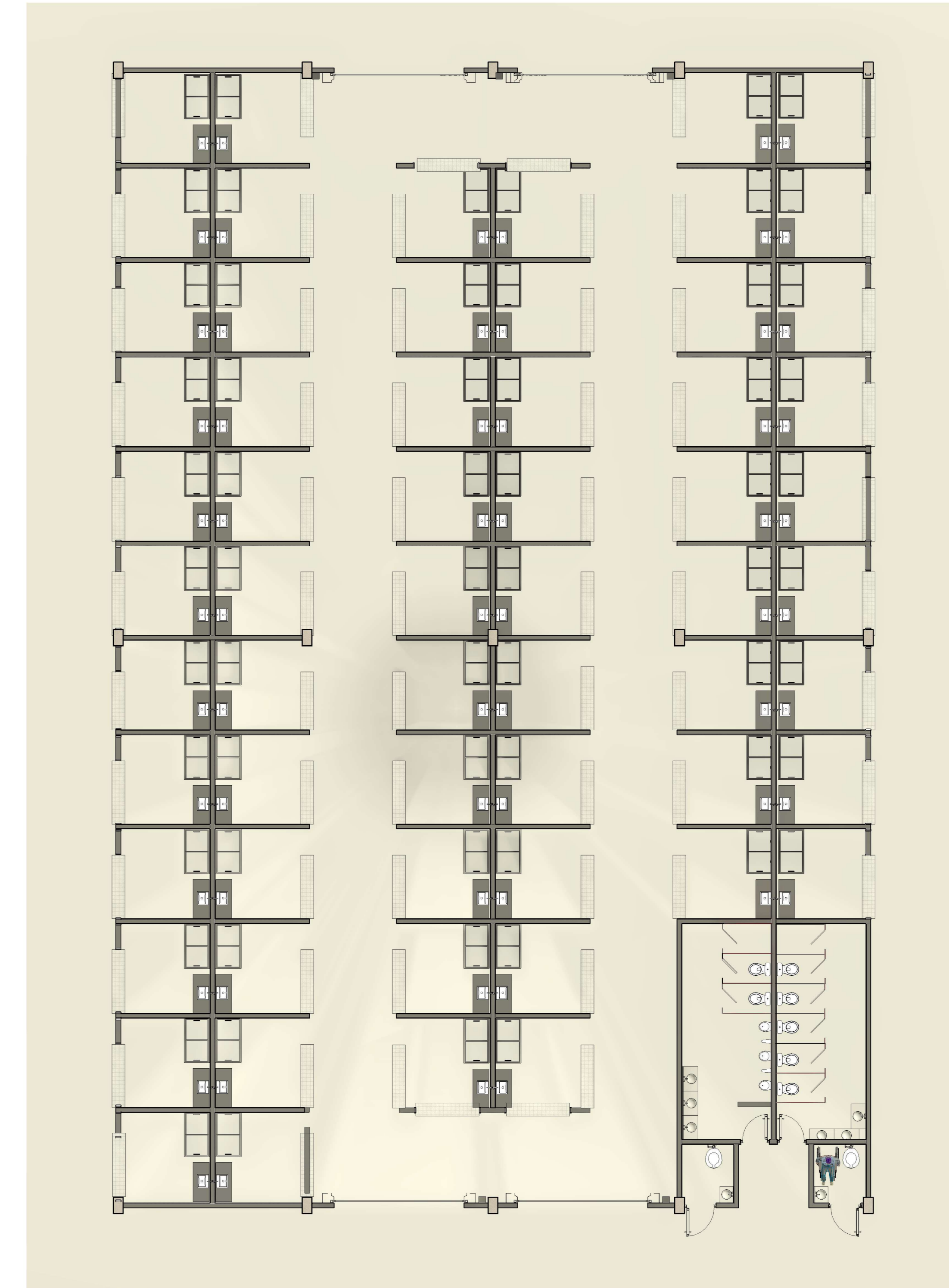
2 TÉRREO 1 : 100
