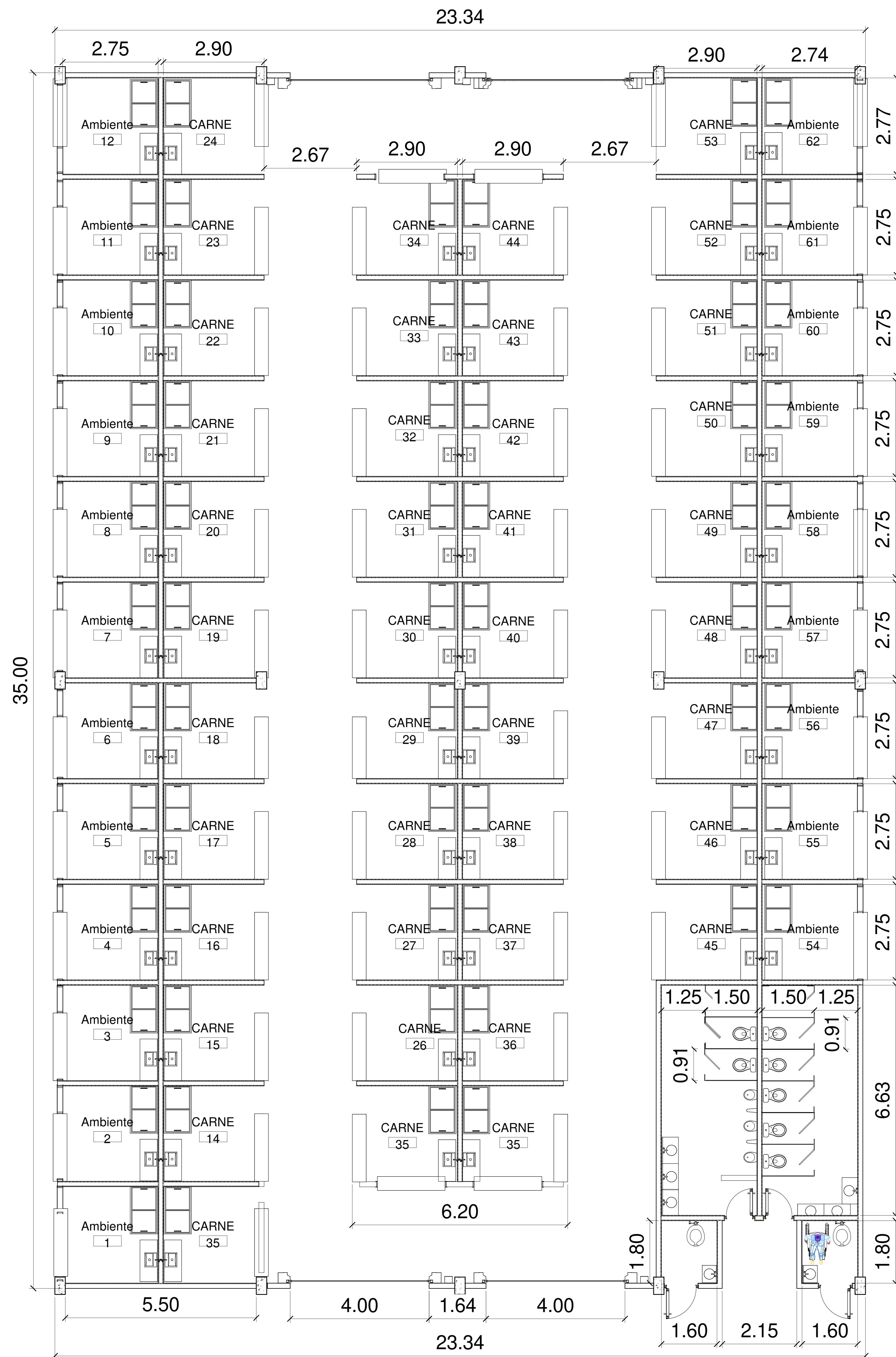
1 PLANTA BAIXA 1 : 50
