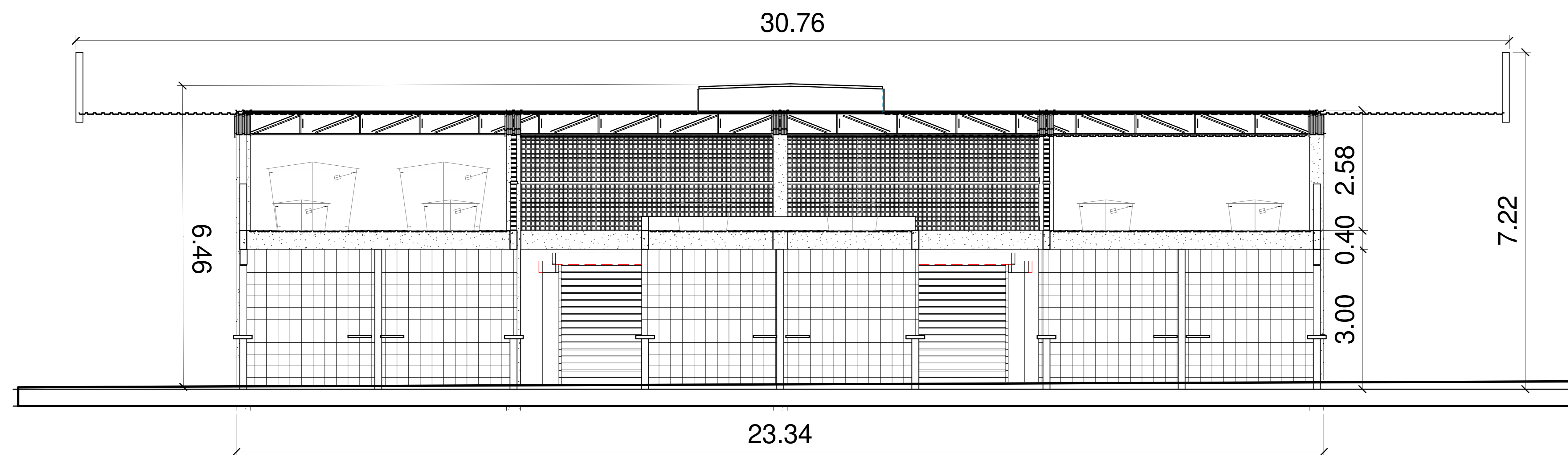
1 CORTE BB 1:50
