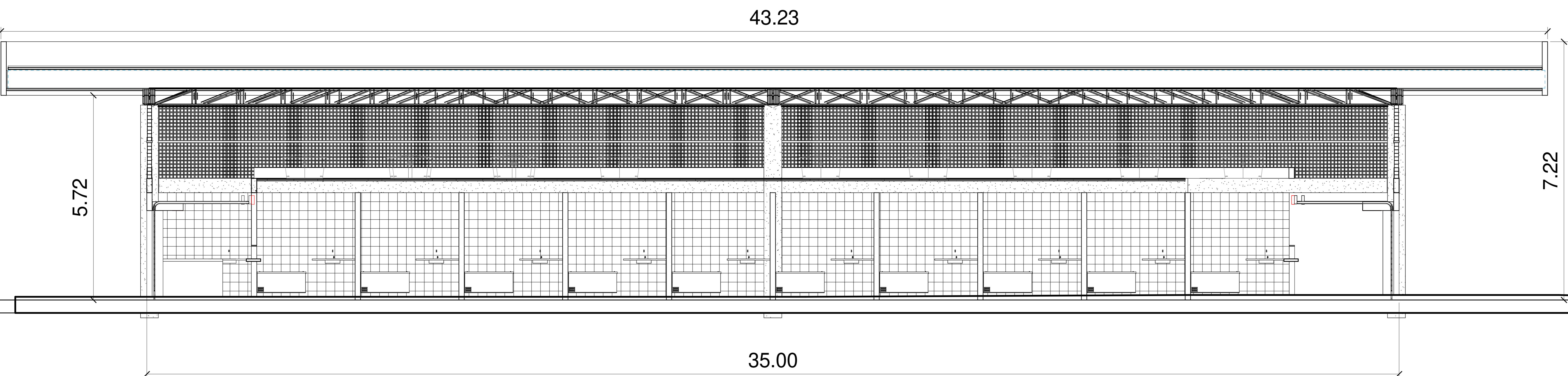
4 CORTE AC 1:50
