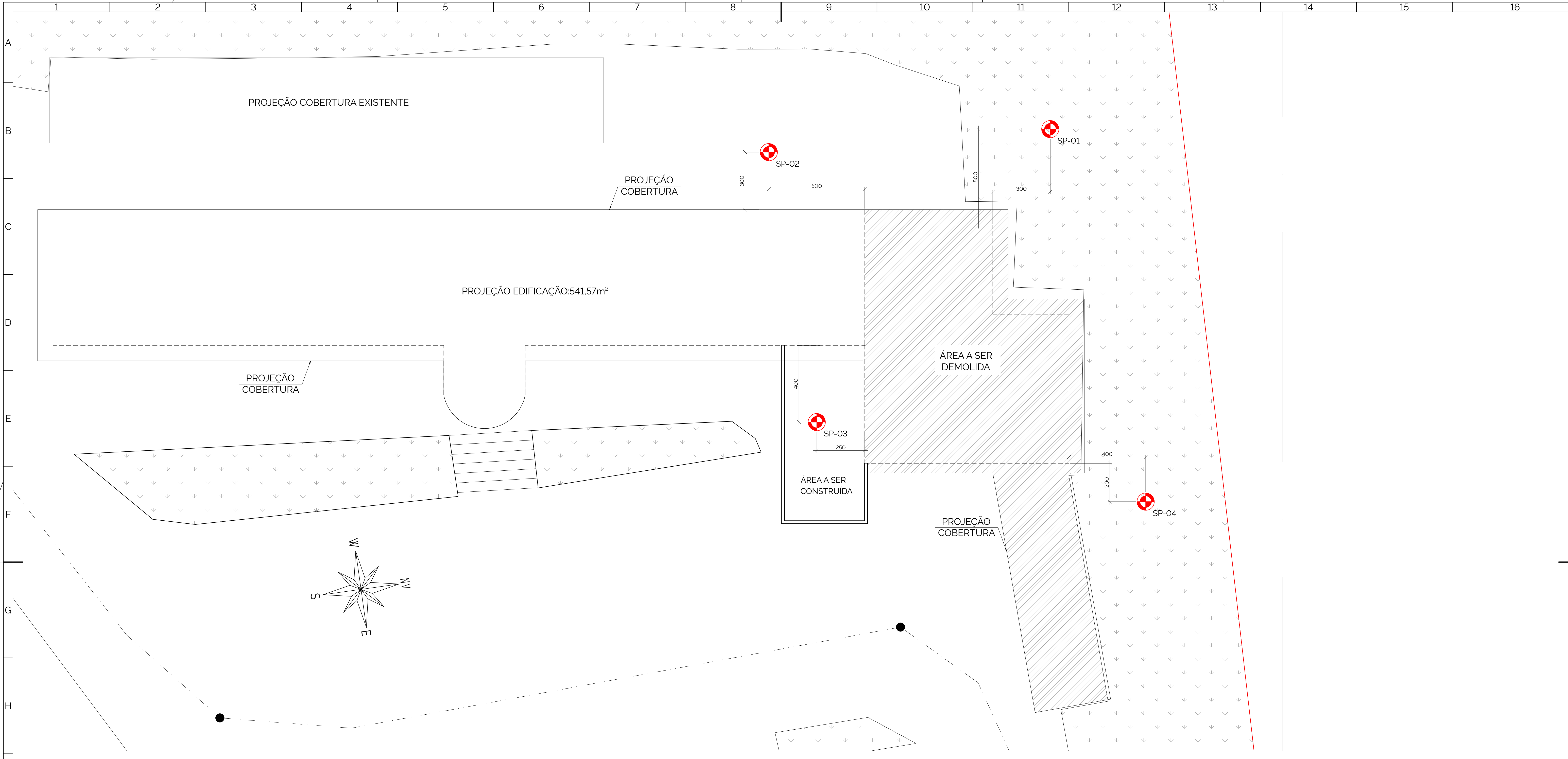
A PLANTA DE LOCAÇÃO DOS FUROS DE SONDAGEM ESC.1:100
