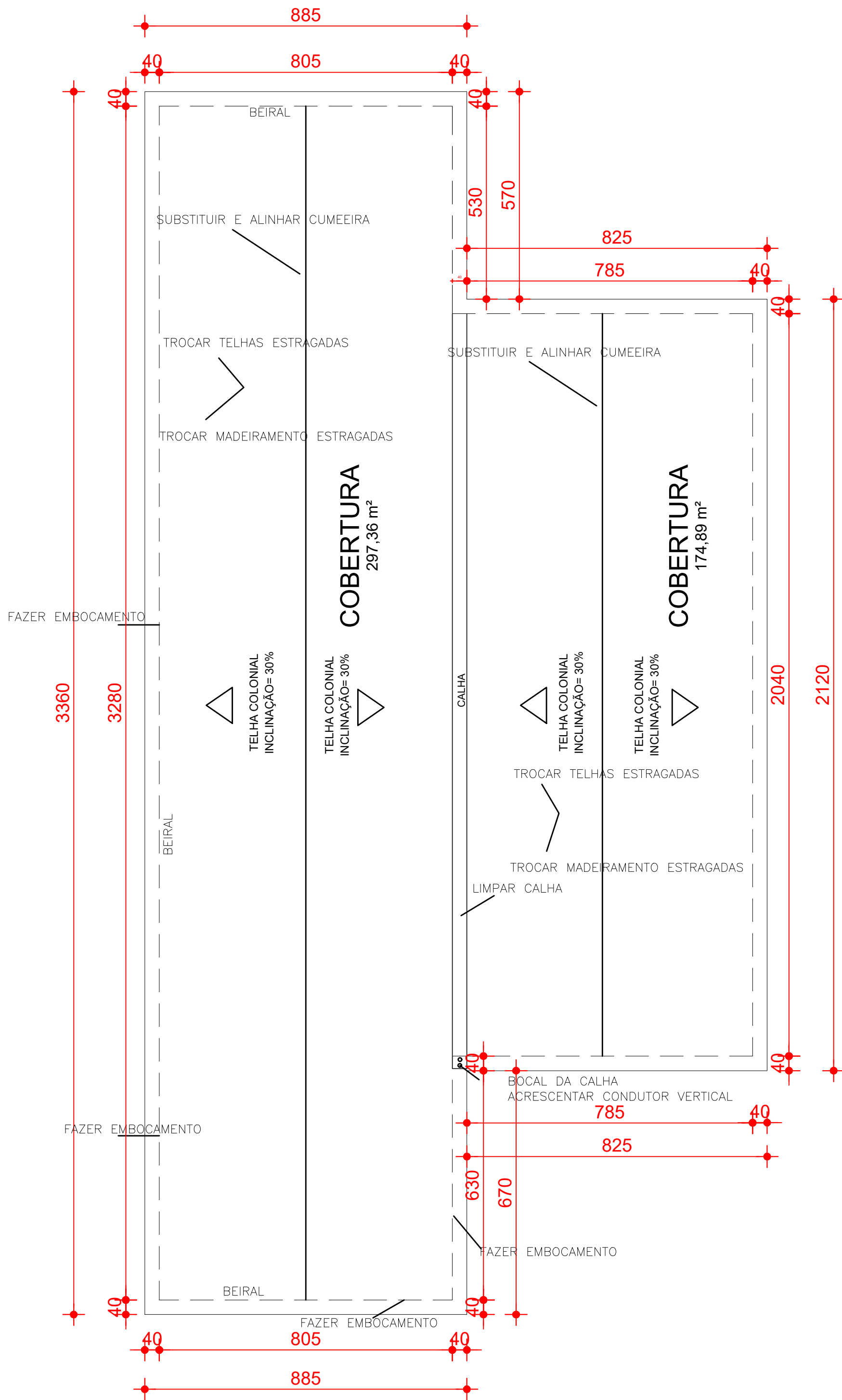
PLANTA EXECUTIVA ESCALA: 1:100
