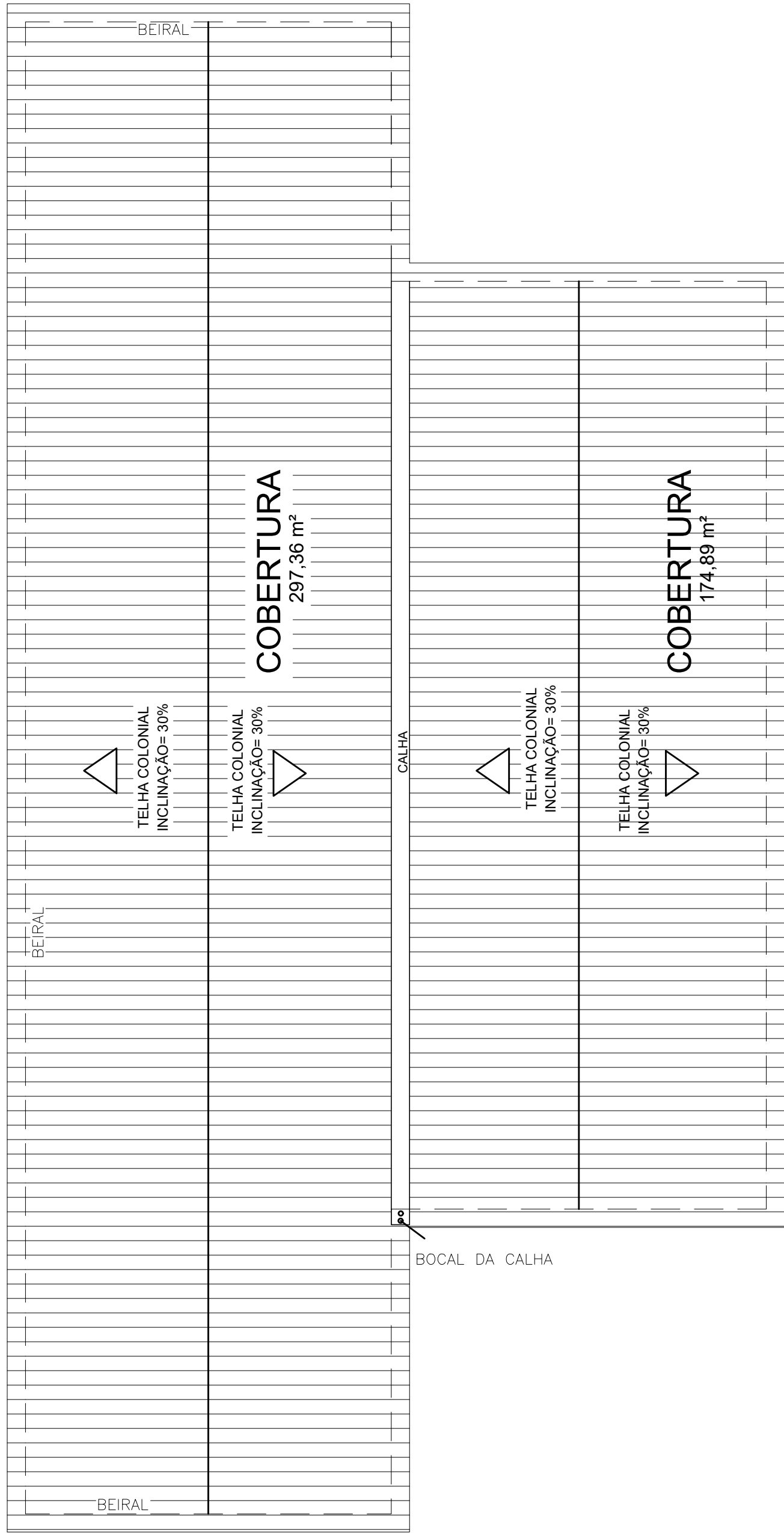
DIAGRAMA DE COBERTURA ESCALA: 1:100
