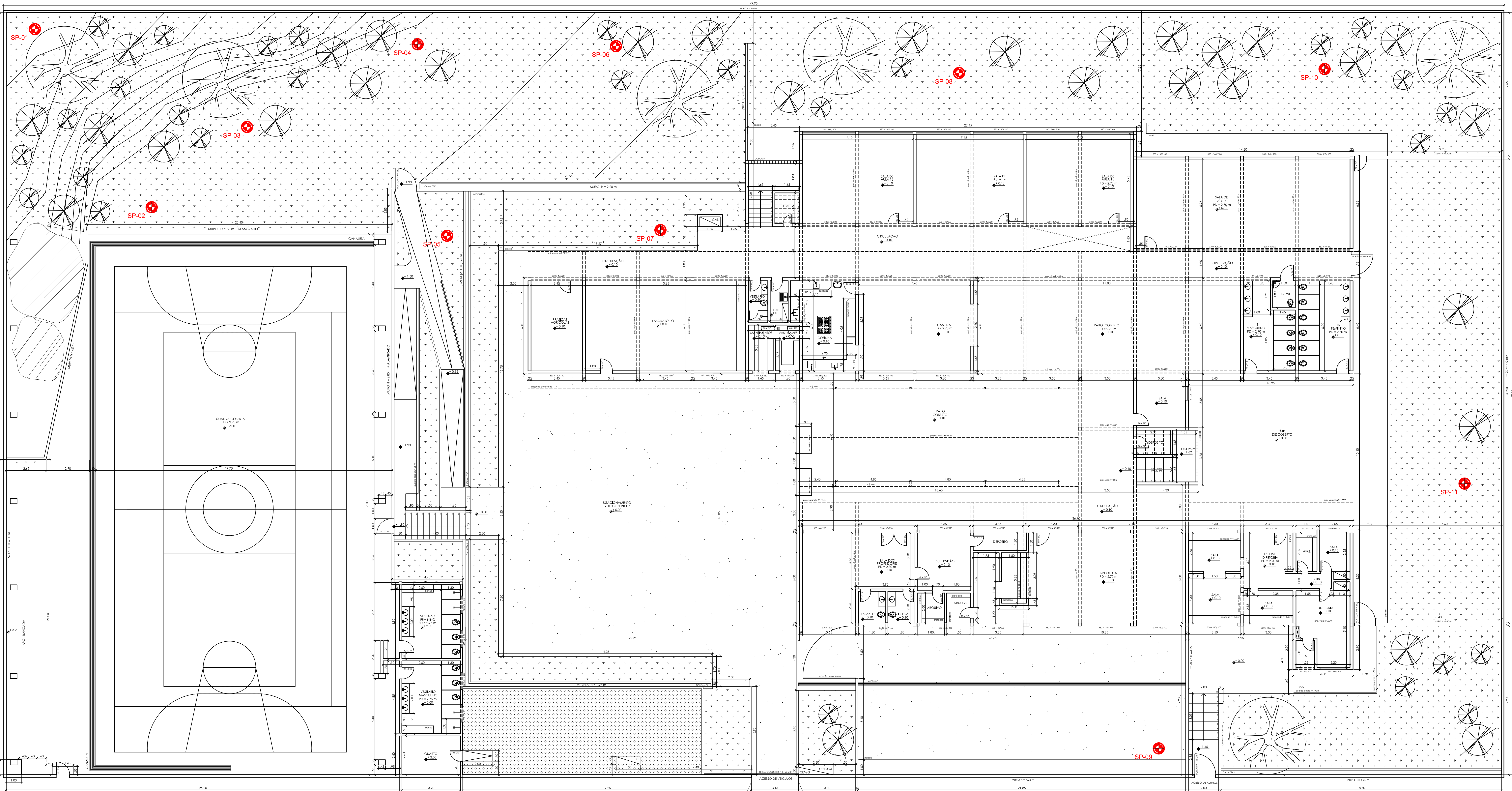
PLANTA 1º PAVIMENTO ESCALA 1/50
