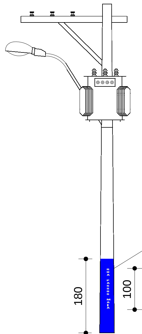
VISTA LATERAL PINTURA POSTES SEM ESCALA
