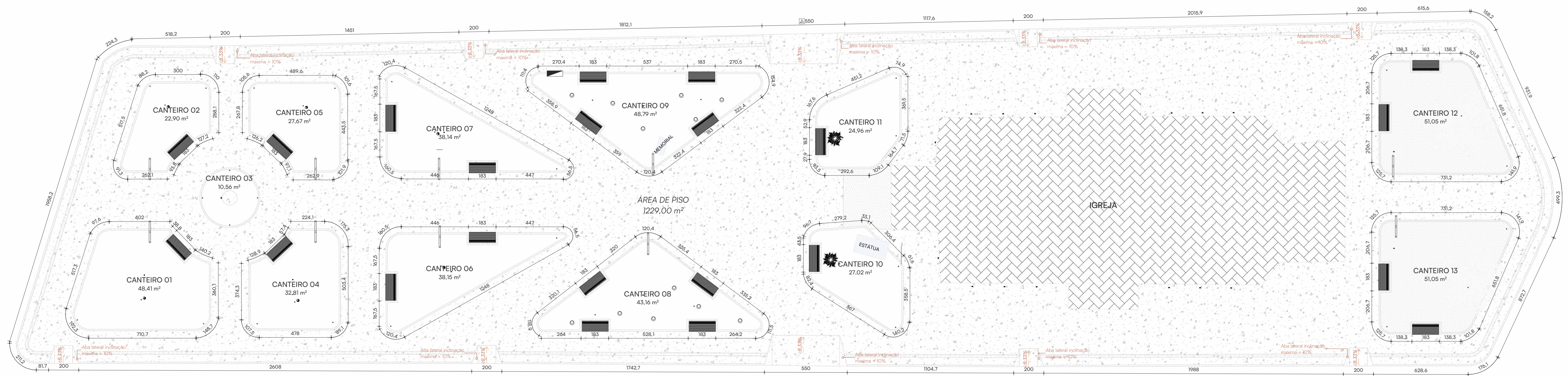
01 PLANTA TÉCNICA - TÉRREO Escala: 1 : 150
