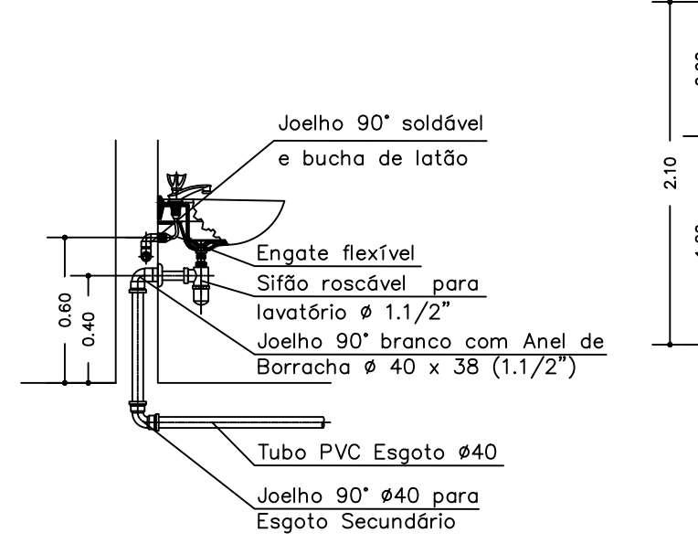
LAVATÓRIO SEM ESCALA
