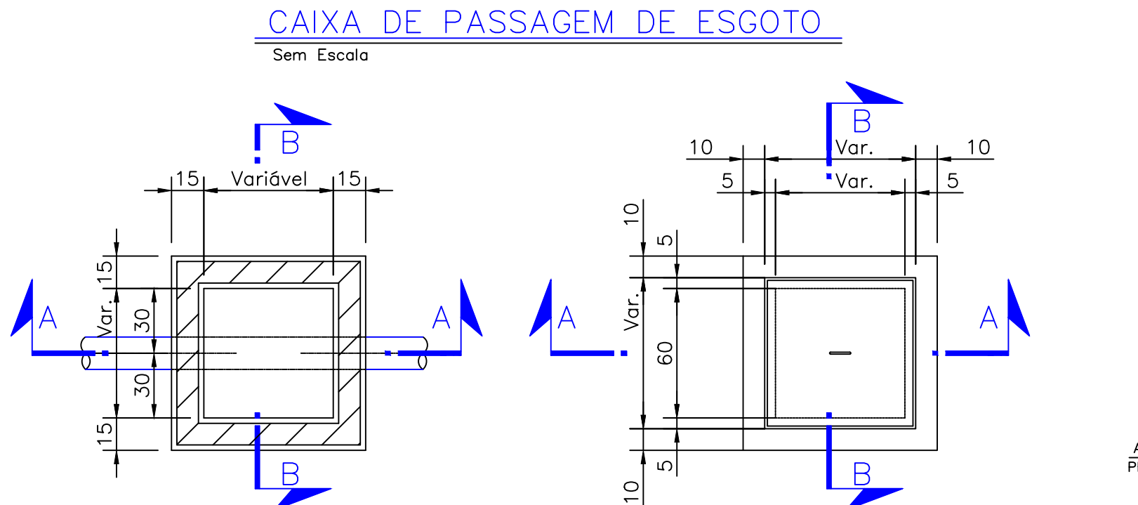
CAIXA DE PASSAGEM DE ESGOTO Sem Escala
