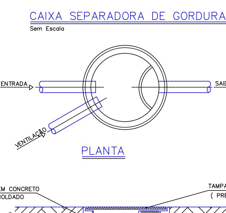
CAIXA SEPARADORA DE GORDURA Sem Escala
