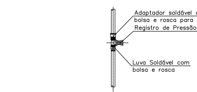
REGISTRO DE PRESSÃO (AF) ACABAMENTO CROMADO SEM ESCALA
