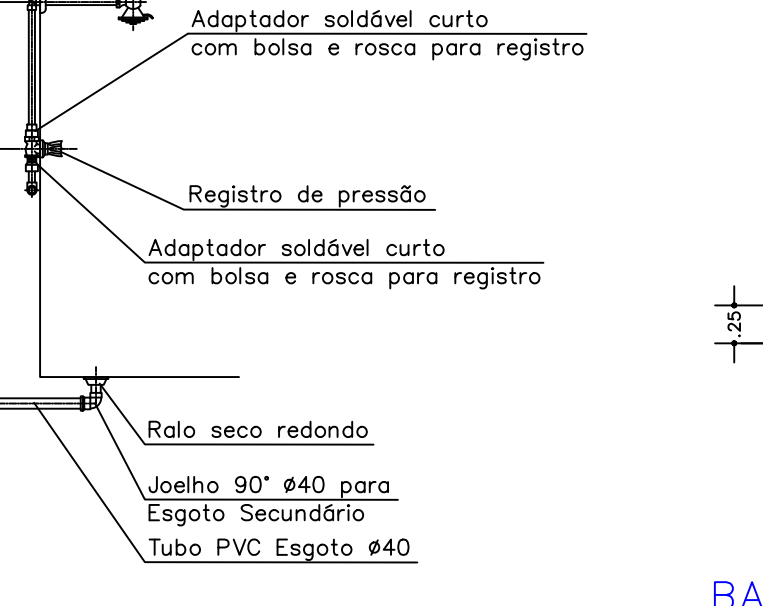
CHUVEIRO SEM ESCALA
