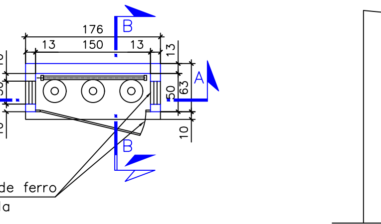
PLANTA
