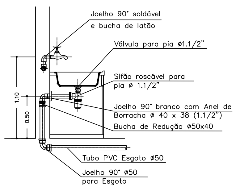
PIA DE COZINHA SEM ESCALA
