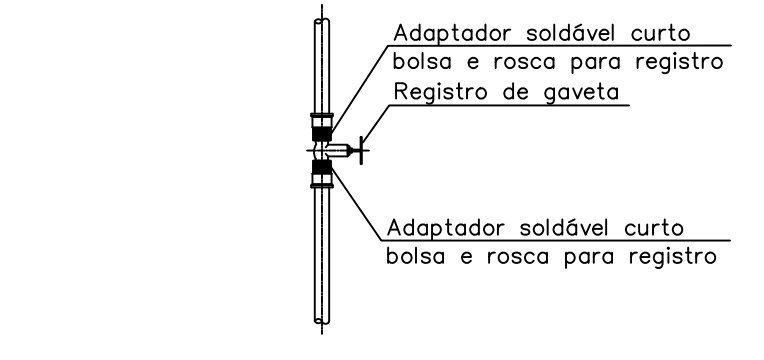
REGISTRO DE GAVETA (AF) ACABAMENTO BRUTO SEM ESCALA
