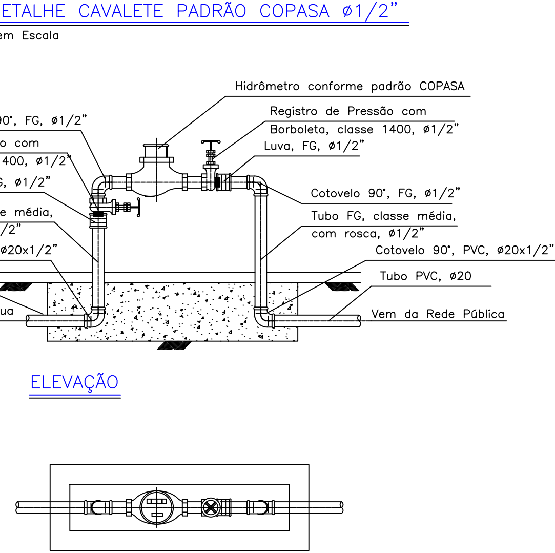
DETALHE CAVALETE PADRÃO COPASA Ø1/2"
