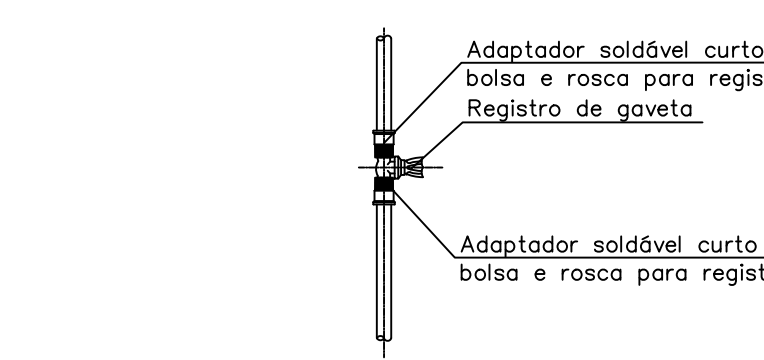
REGISTRO DE GAVETA (AF) ACABAMENTO CROMADO SEM ESCALA
