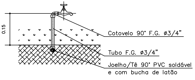
TORNEIRA DE JARDIM SEM ESCALA
