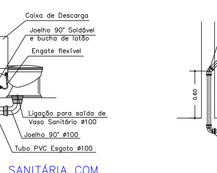
BACIA SANITÁRIA COM CAIXA ACOPLADA SEM ESCALA
