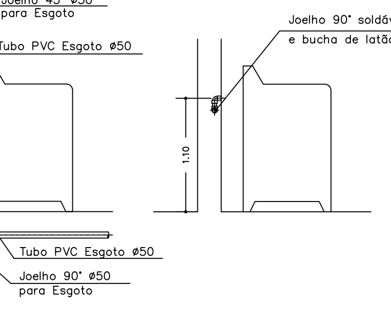
MÁQUINA DE LAVAR ROUPA SEM ESCALA
