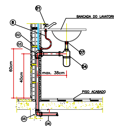
LIGAÇÃO DO LAVATÓRIO DE BANCADA VISTA LATERAL - SEM ESCALA
