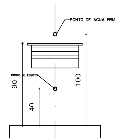
LIGAÇÃO DO TANQUE VISTA FRONTAL - SEM ESCALA
