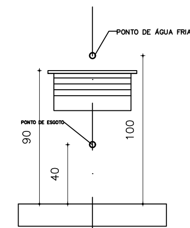
LIGAÇÃO DO TANQUE VISTA FRONTAL - SEM ESCALA
