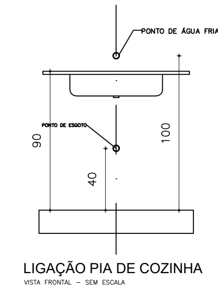
LIGAÇÃO PIA DE COZINHA VISTA FRONTAL - SEM ESCALA
