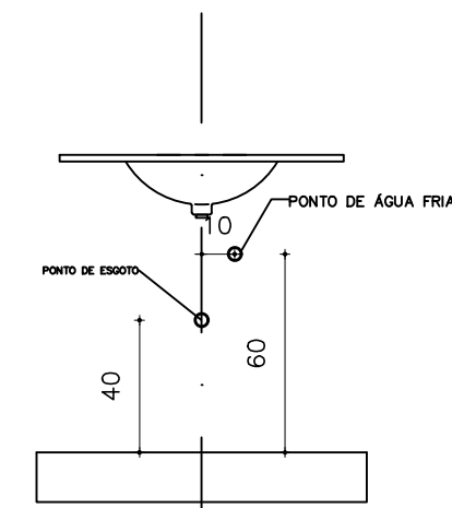
LIGAÇÃO DO LAVATÓRIO DE BANCADA VISTA FRONTAL - SEM ESCALA
