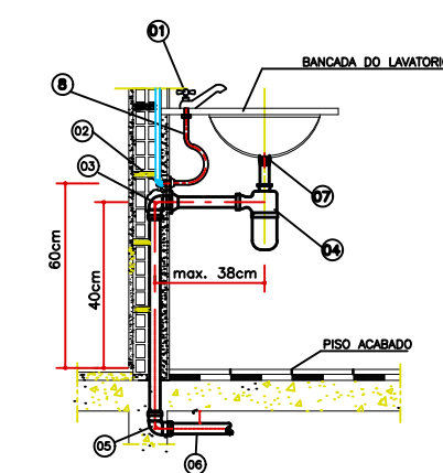
LIGAÇÃO DO LAVATÓRIO DE BANCADA VISTA LATERAL - SEM ESCALA
