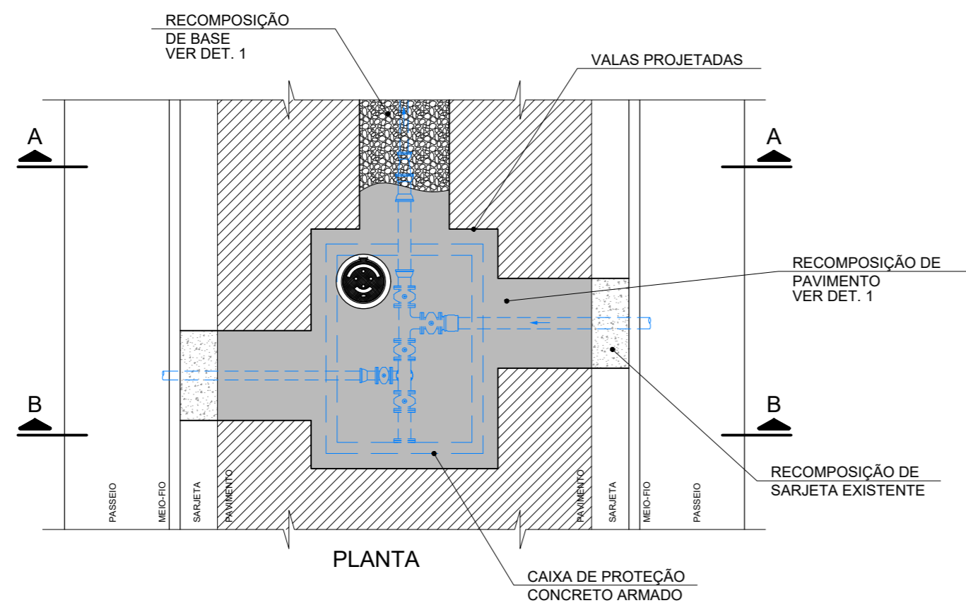
DETALHE DE RECOMPOSIÇÃO DE VALAS E PAVIMENTO SEM ESCALA
