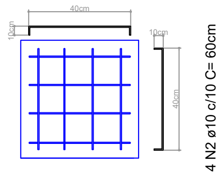
PLANTA ESC 1:25
