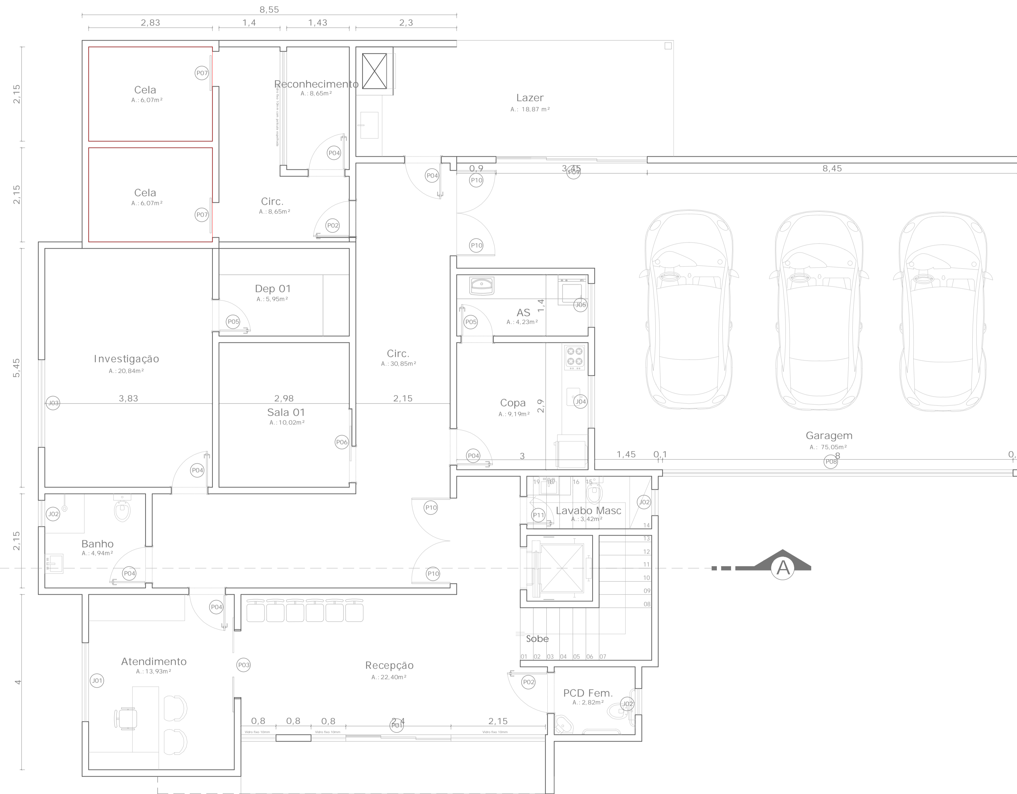
Planta Baixa Térreo (291,19m²) Esc.: 1/50
