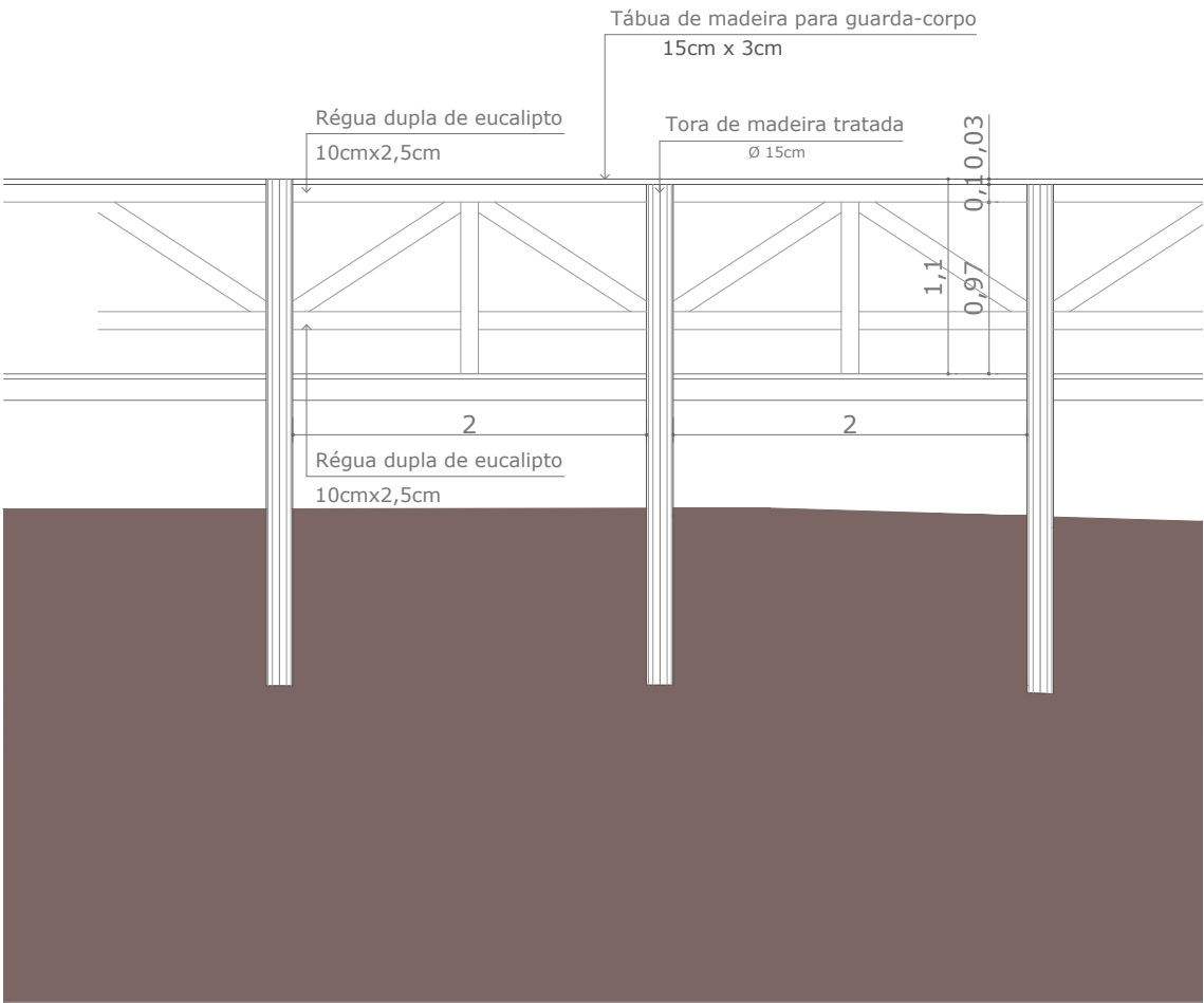
Detalhe Guarda-corpo Esc.:1/40
