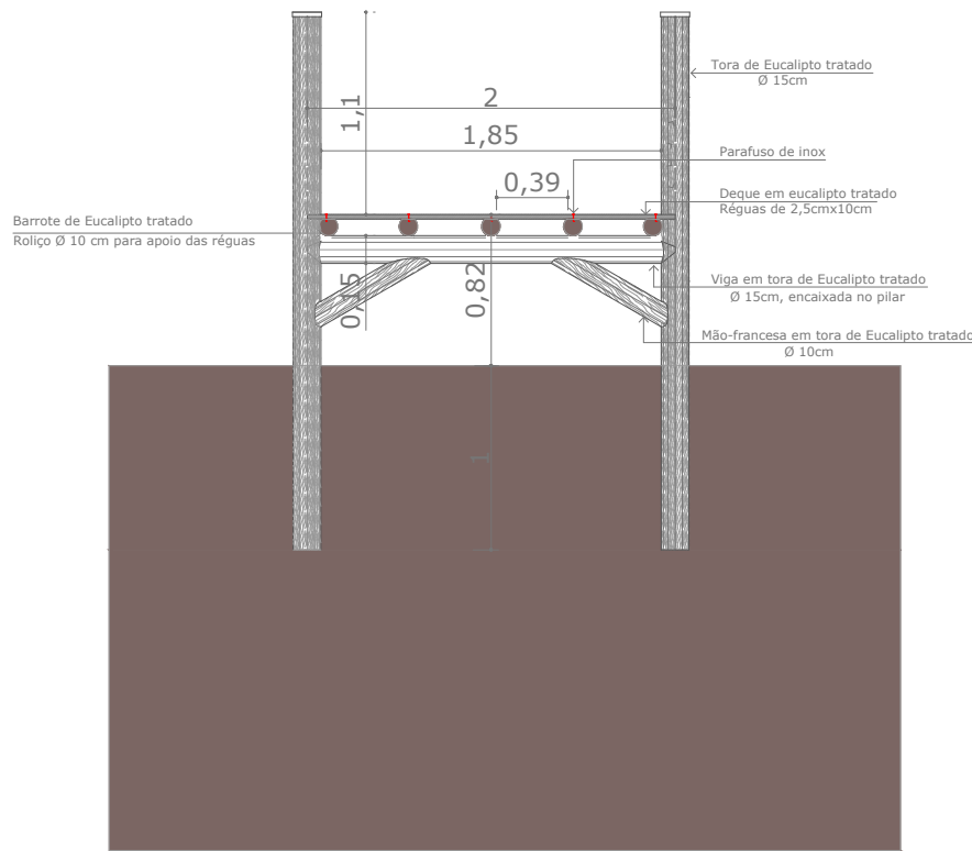
Corte AA Esc.:1/40
