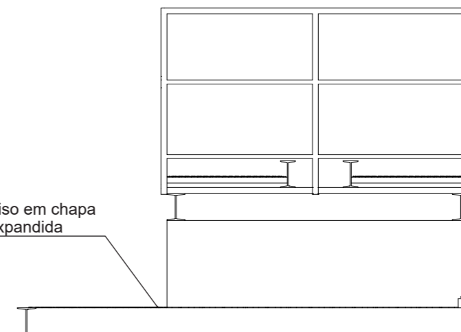
Vista Lateral 1:50
