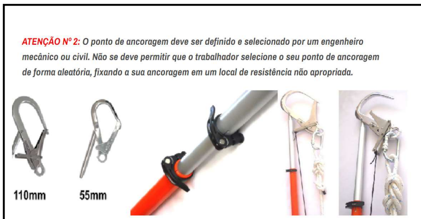
Vara de manobra extensiva para ancoragem de segurança do trabalho em altura.
