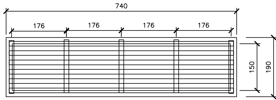
CAIXA COLETORA 01 e 02 ESCALA: 1/75
