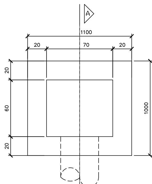
PLANTA - BOCA DE LOBO
