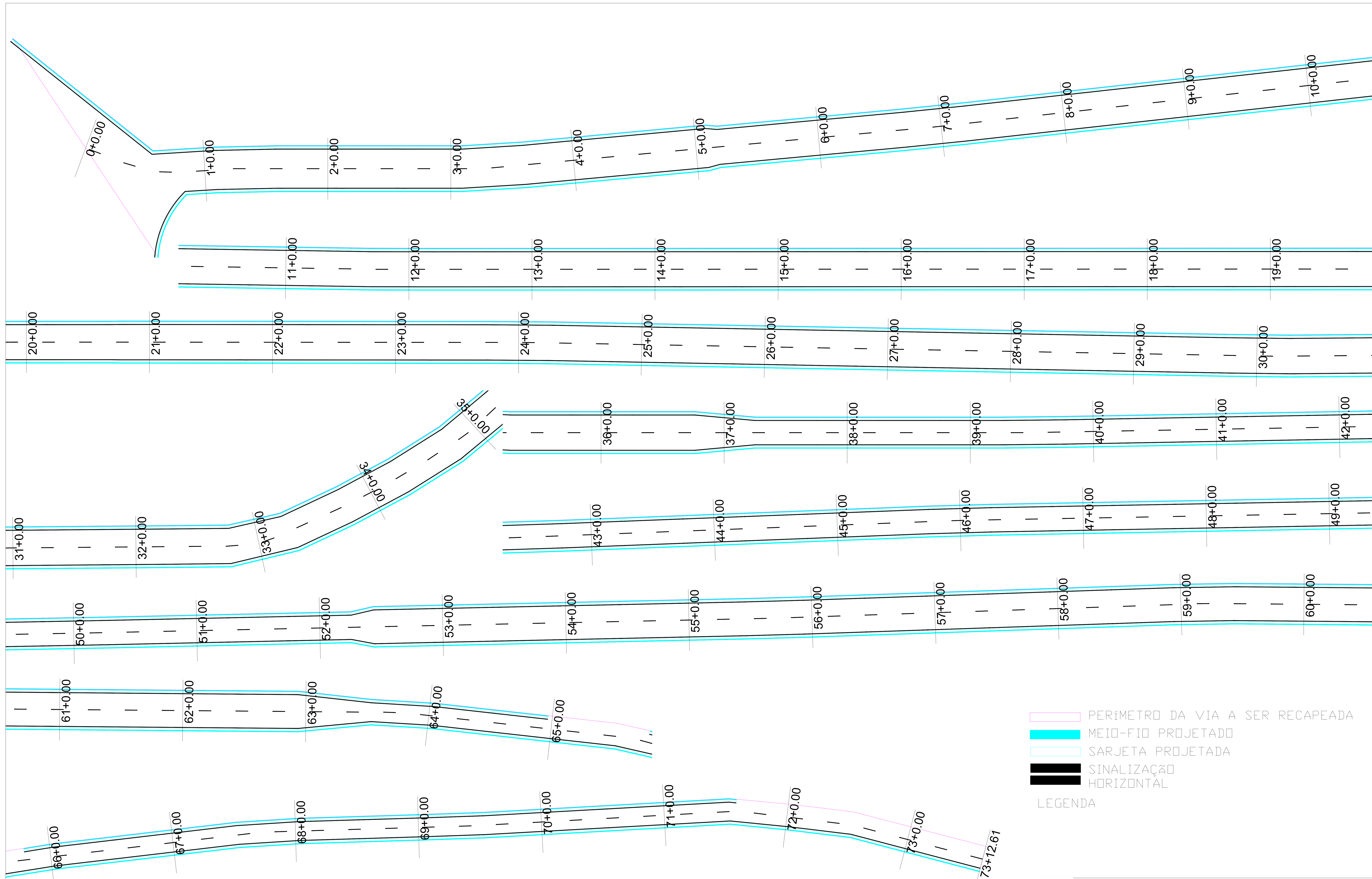
PLANTA DE RECAPEAMENTO E SINALIZAÇÃO ESTACA 0 À 73+12,61 ESCALA=1:5000
